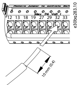
Illustration 5.19 Raccordement de fils de commande solides
