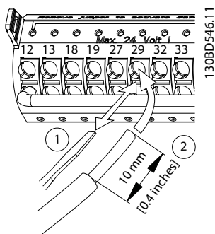
Illustration 5.20 Raccordement de fils de commande flexibles
