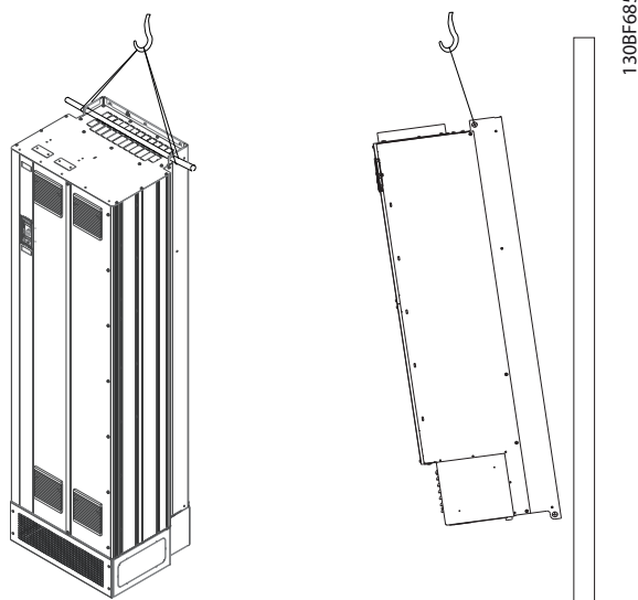
Illustration 4.2 Méthode de levage recommandée
