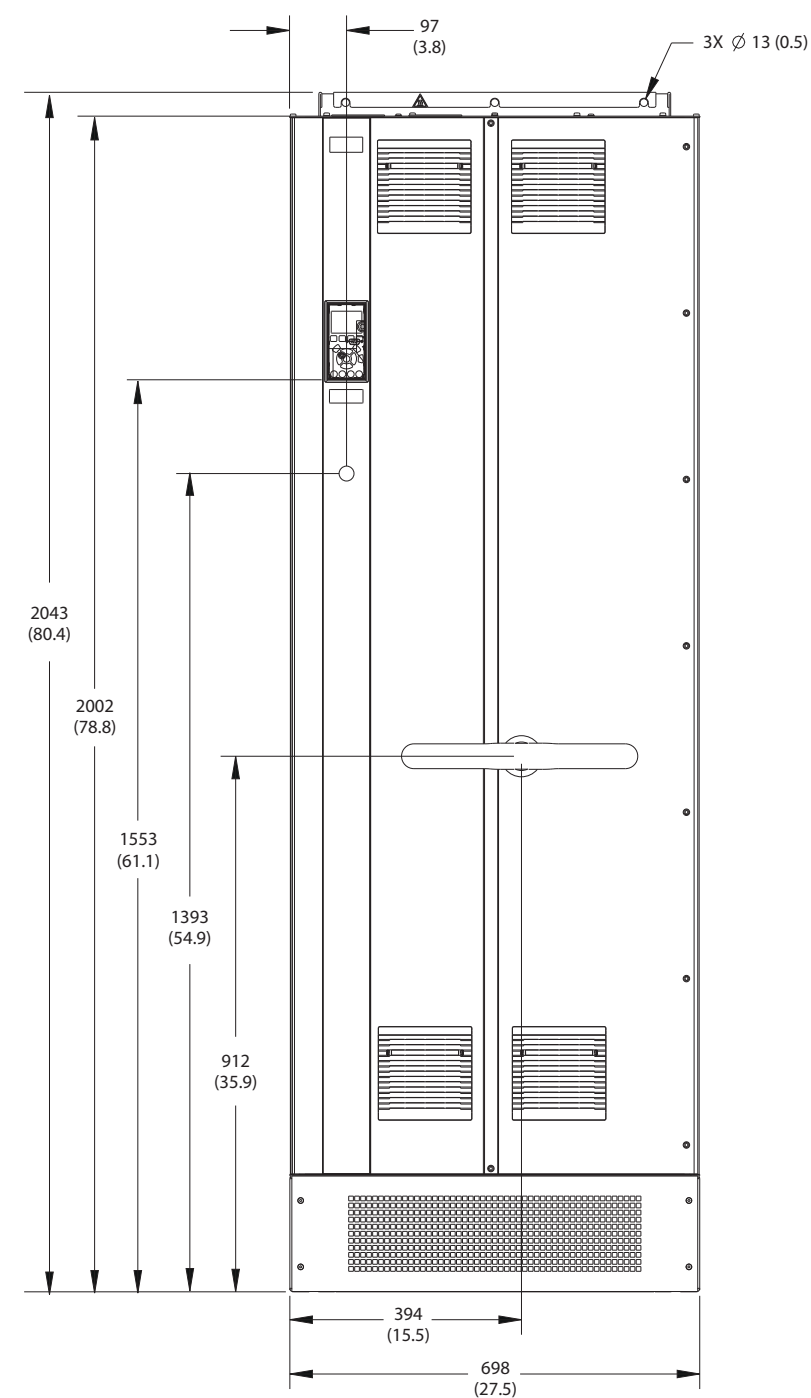
Illustration 9.6 Vue frontale du boîtier E2h
