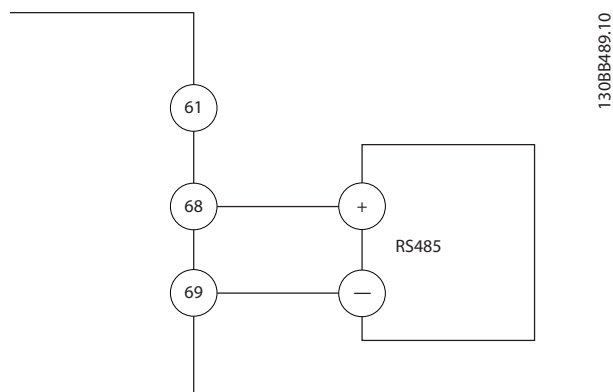
Illustration 5.21 Schéma de câblage de la communication série
