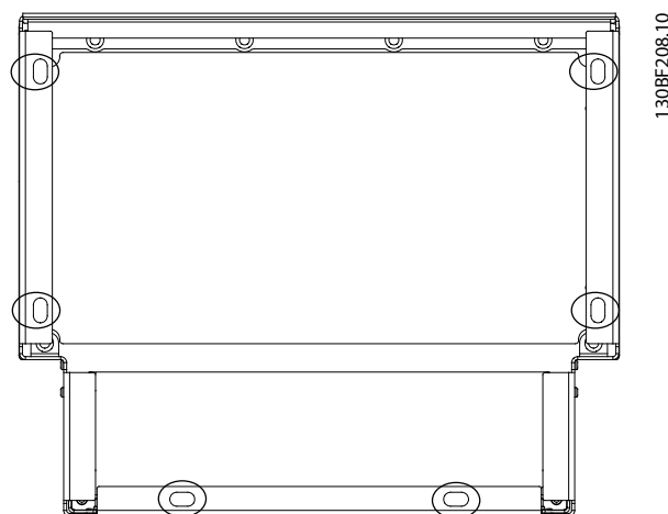
Illustration 4.3 Points de fixation au sol du socle
