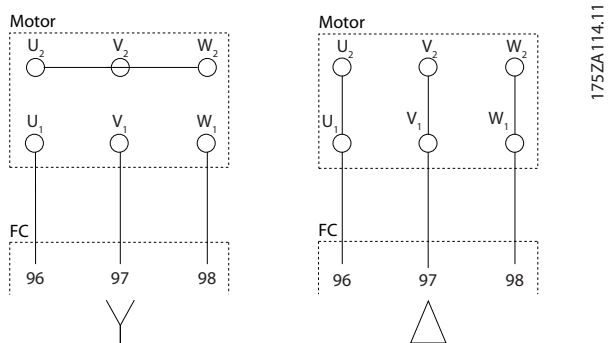
Illustration 4.2 Connexions en étoile et en triangle
