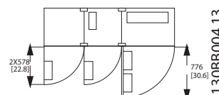
Illustration 3.14 Espace devant la protection nominale IP21/IP54 type F3
