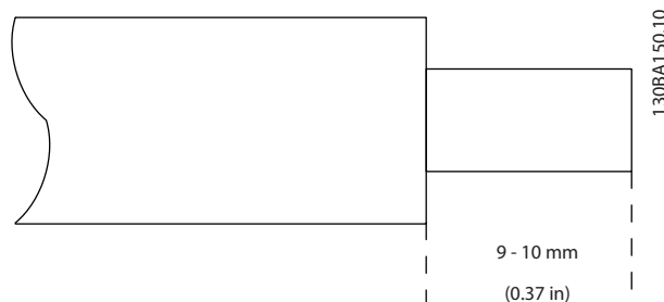
Illustration 4.17 Dénuder l'isolant
