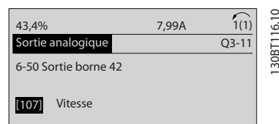
Illustration 6.8 Réglage d'un paramètre
