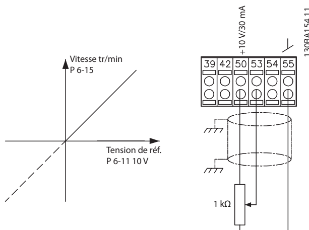
Illustration 4.30 Référence potentiomètre
