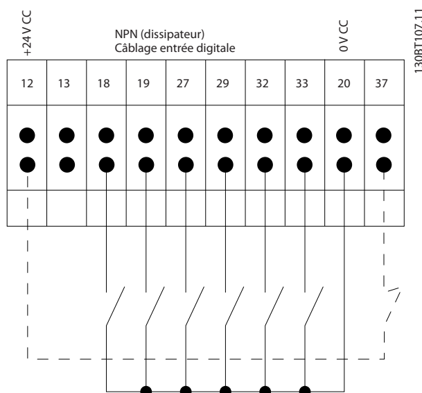
Illustration 4.24 Polarité NPN
