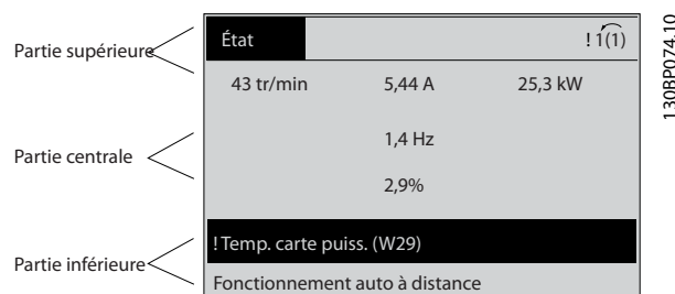
Illustration 5.5 Sections d'affichage
