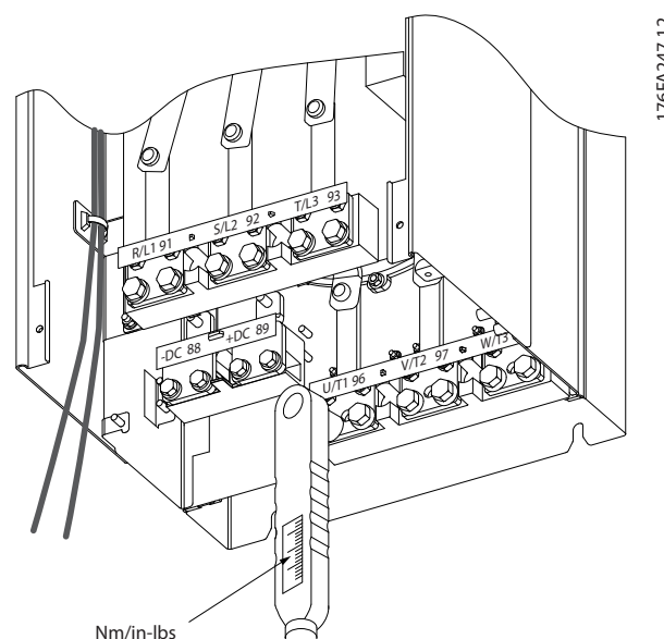
Illustration 4.10 Serrer les boulons avec une clé dynamométrique
