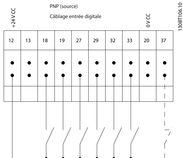
Illustration 4.23 Polarité PNP
