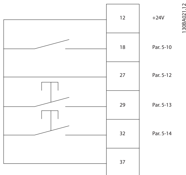
Illustration 4.29 Accélération/décélération
