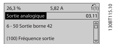
Illustration 6.7 Paramètre 6-50 S.born.42 sélectionné
