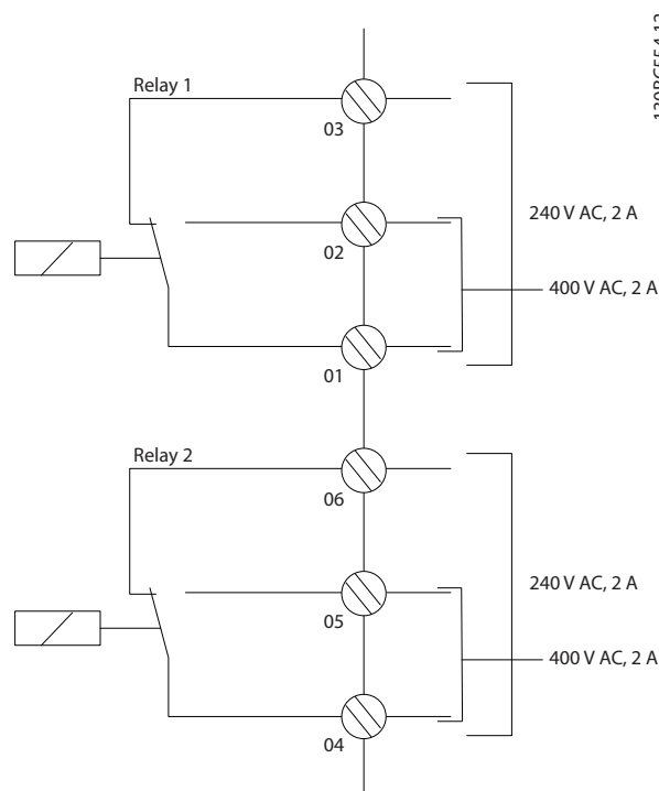
Illustration 5.12 Sorties relais supplémentaires
