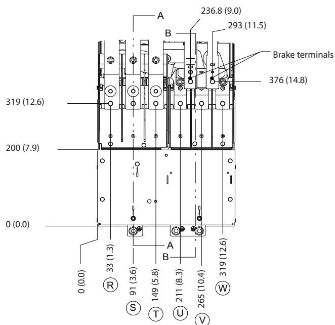
Illustration 7.3 Dimensions des bornes du module de variateur (Vue de face)
