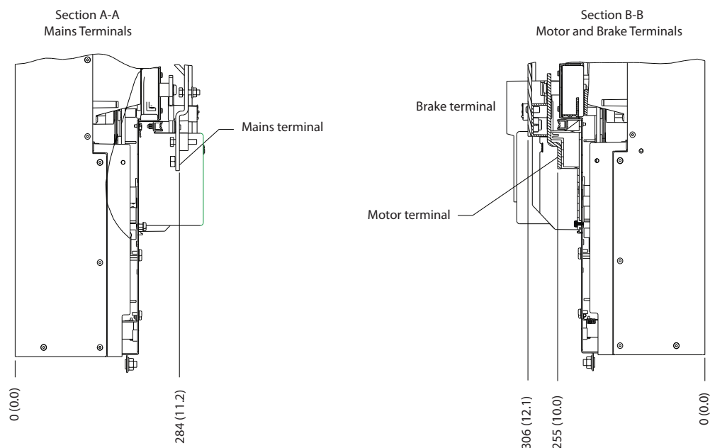
Illustration 7.4 Dimensions des bornes du module de variateur (Vues latérales)
