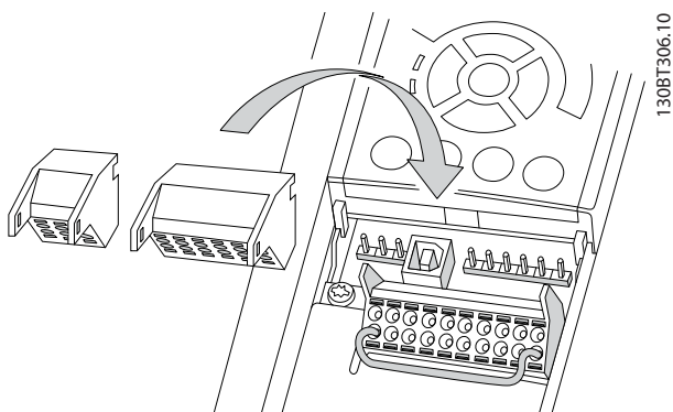
Illustration 5.10 Retrait des bornes de commande
