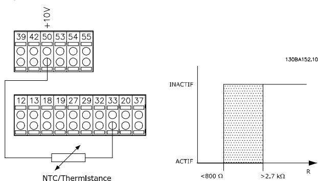
Illustration 5.3 Connexion de la thermistance PTC - Entrée numérique avec alimentation 10 V
