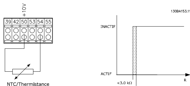
Illustration 5.4 Connexion de la thermistance PTC - Entrée analogique avec alimentation 10 V
