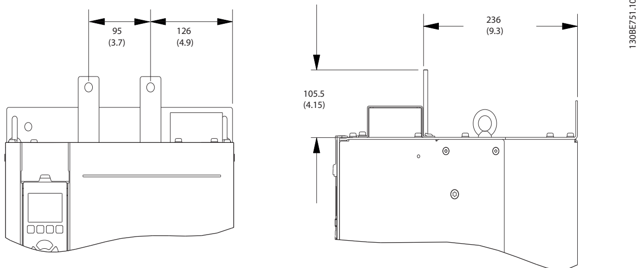
Illustration 7.5 Dimensions du bus CC (vues avant et latérales)
