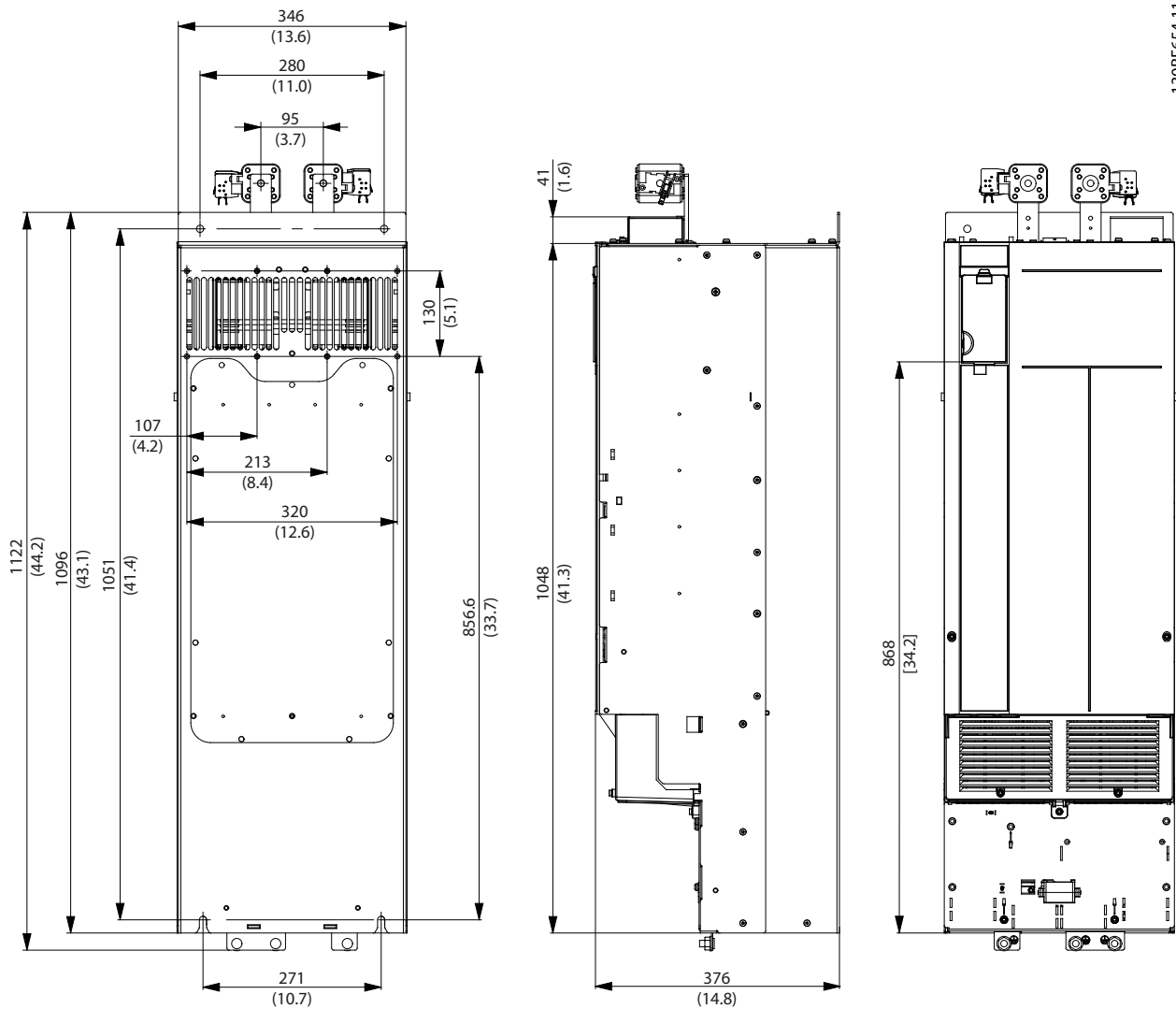
Illustration 7.2 Dimensions d'installation des VLT® Parallel Drive Modules
