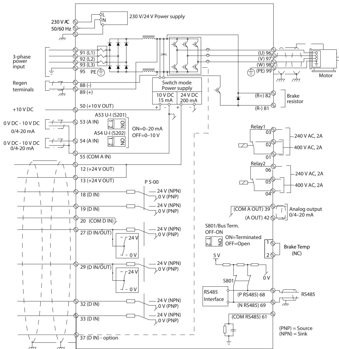
Illustration 5.1 Schéma de câblage
