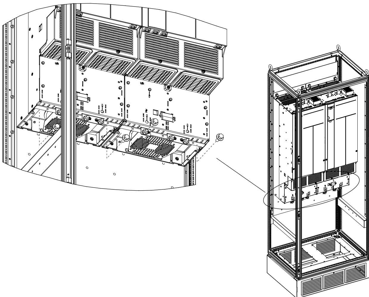
Illustration 4.6 Installation des boulons de montage inférieurs
