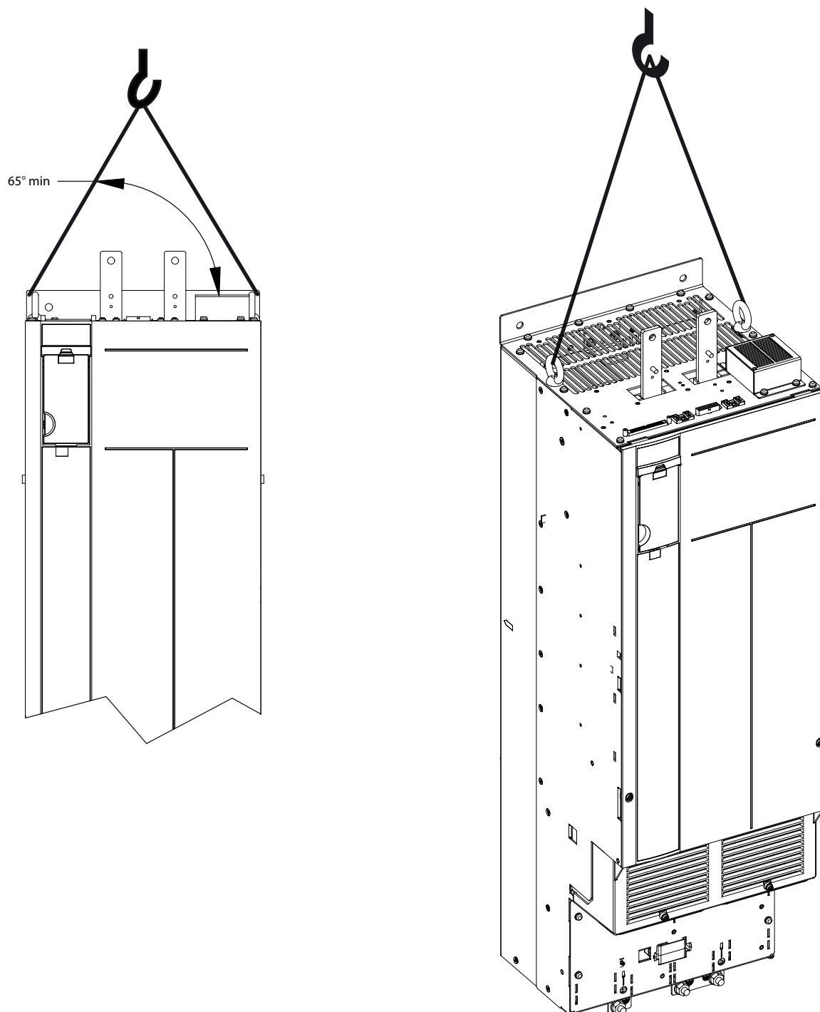
Illustration 4.3 Levage du module de variateur
