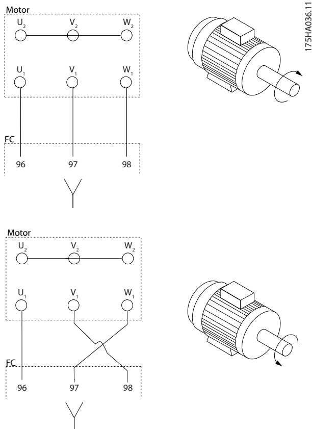
Illustration 5.7 Changement de la rotation du moteur
