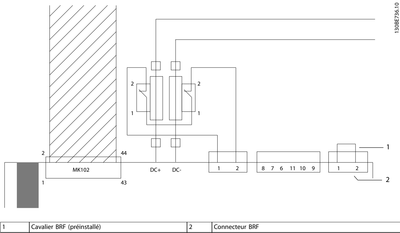
Illustration 8.3 Connexion du cavalier BRF
