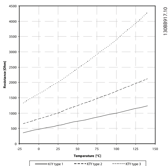
Illustration 5.6 Sélection du type KTY
