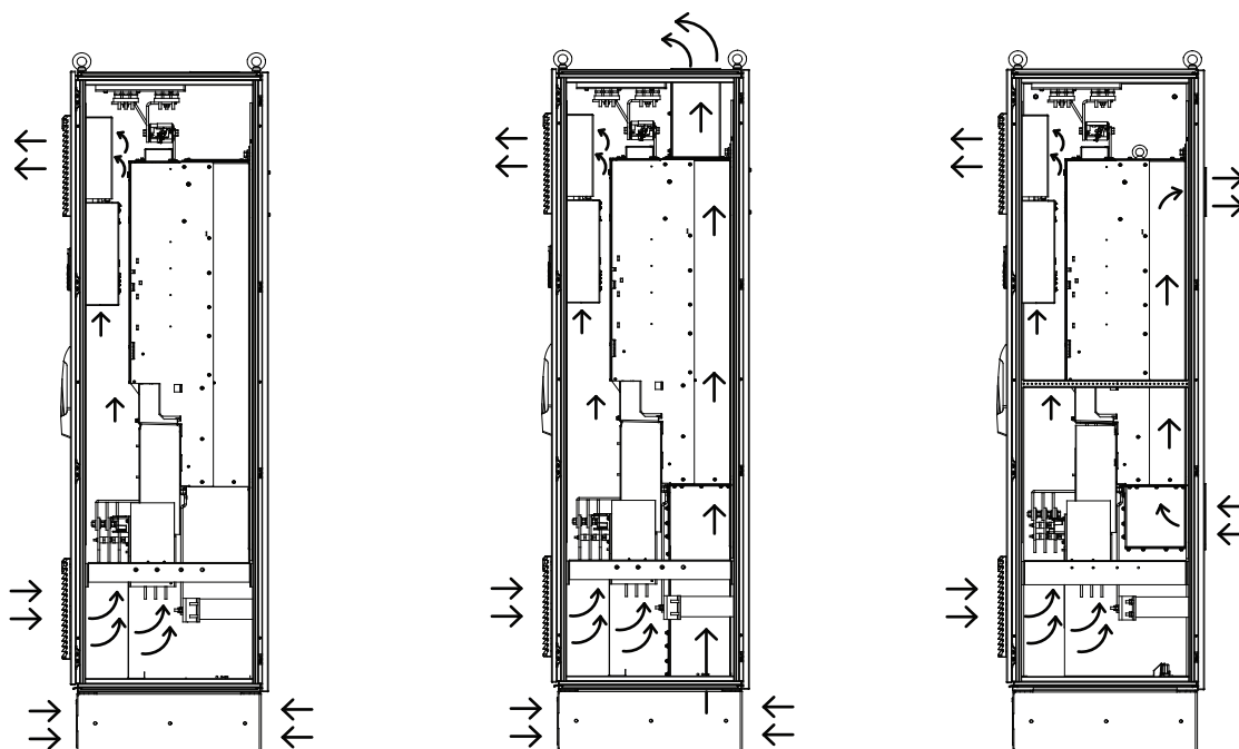
Illustration 4.4 Débit, appareil standard (gauche), kit de refroidissement par le bas/dessus (milieu) et kit de refroidissement par l'arrière (droite)
