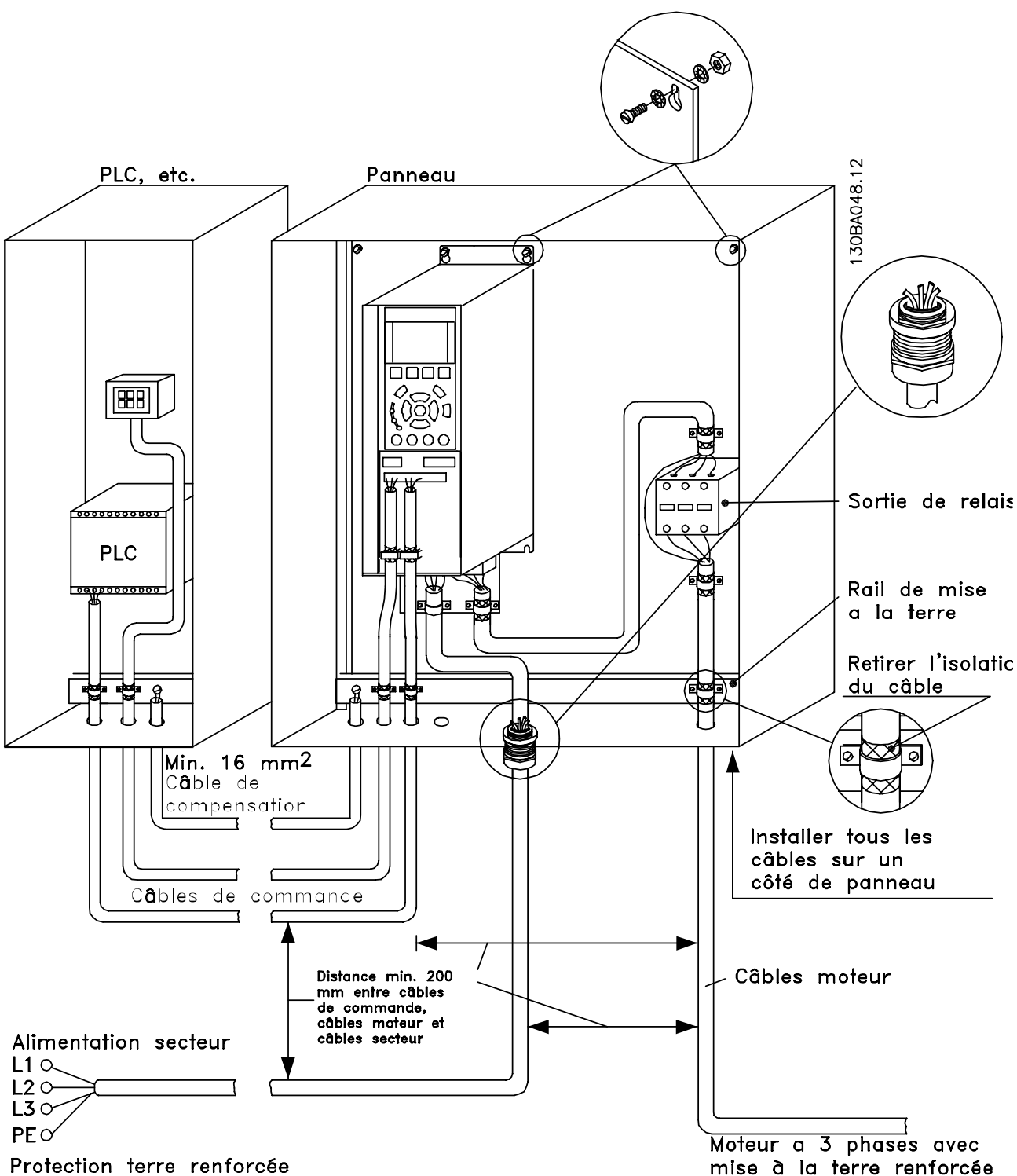
Illustration 5.13 Installation électrique d'un variateur de fréquence dans une armoire conforme aux normes CEM
