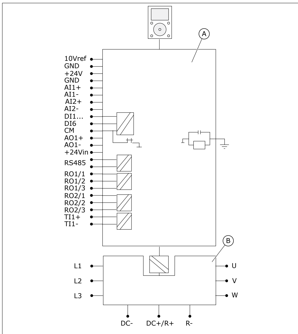
Fig. 25: Les isolations galvaniques
