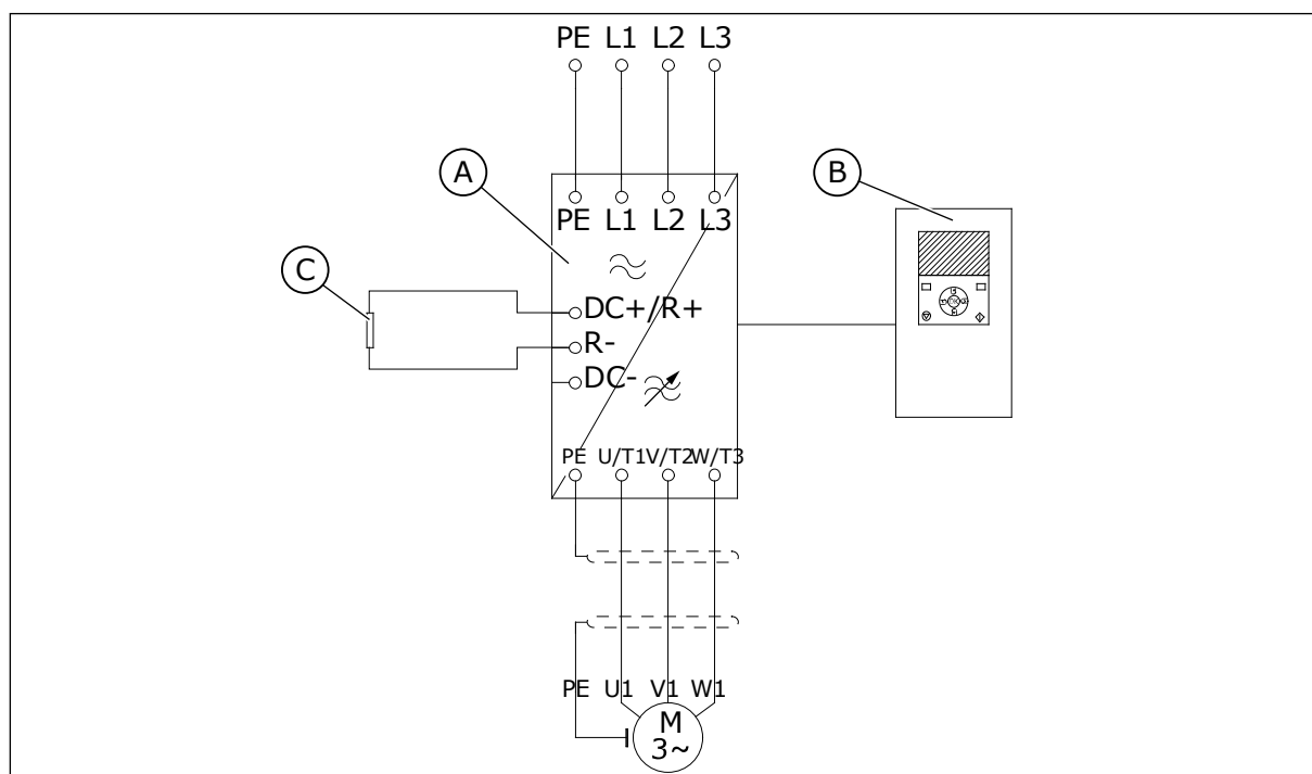
Fig. 8: Schéma général MR8 et MR9
