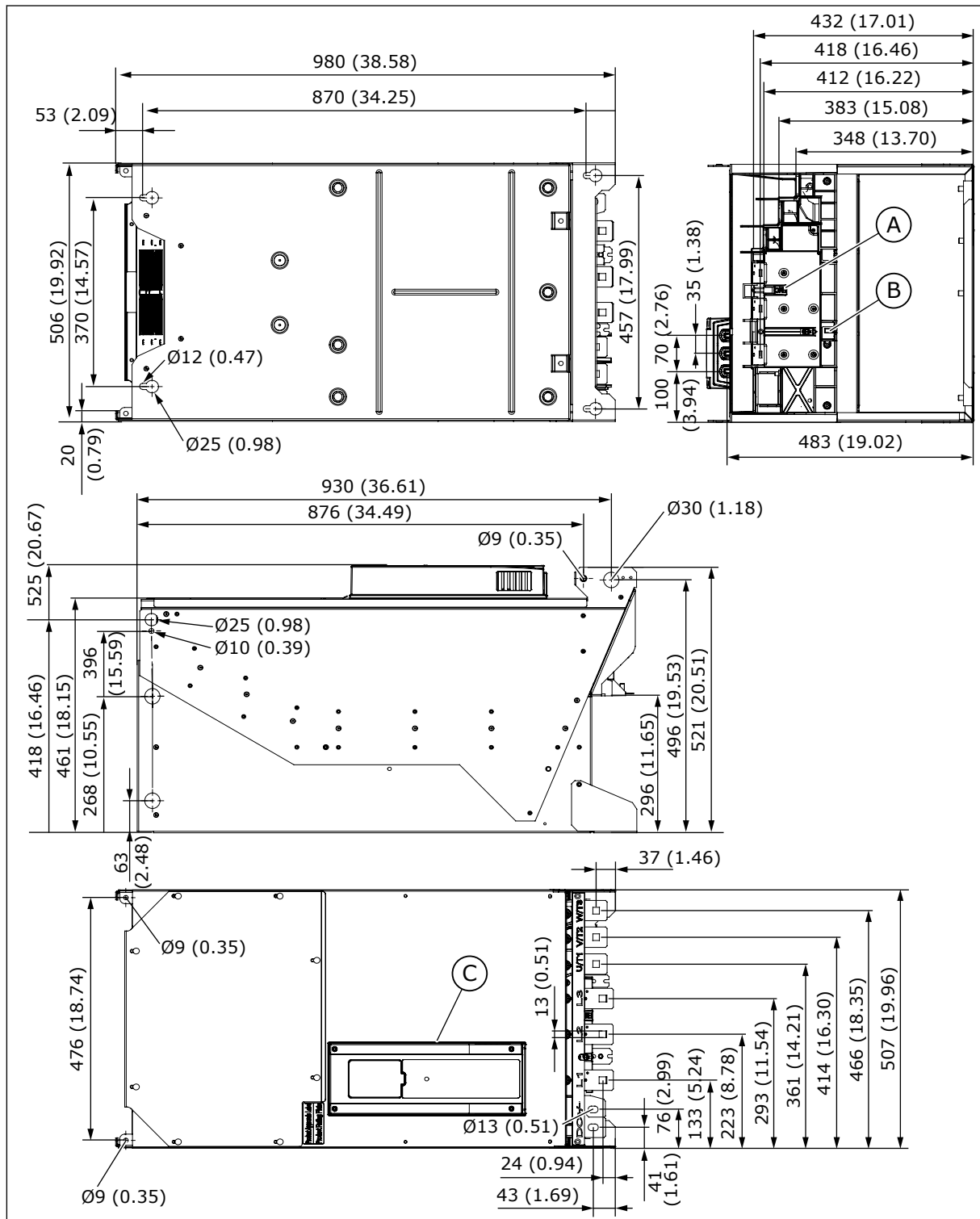
Fig. 5: Dimensions sans le module d'options [mm (pouces)]
