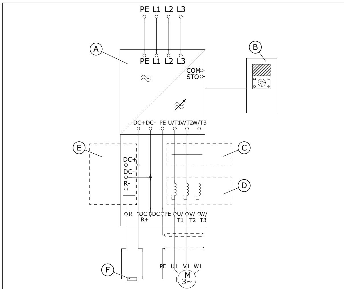
Fig. 10: Schéma général MR10 avec le module d'options
