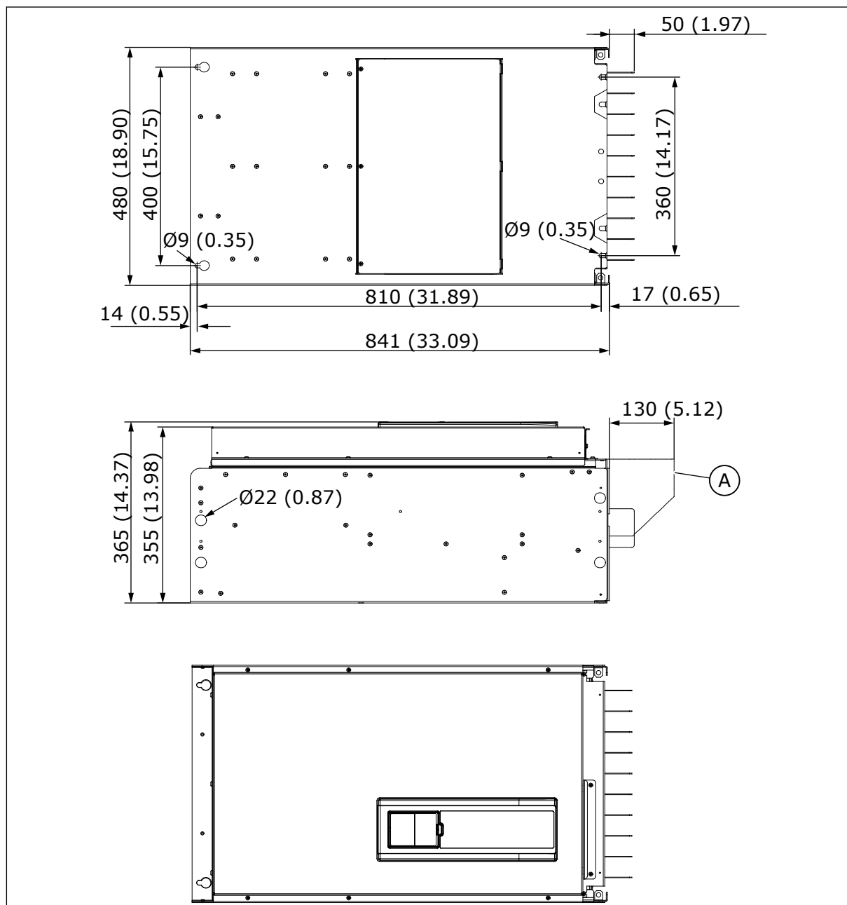
Fig. 4: Dimensions du convertisseur de fréquence, MR9 [mm (pouces)]
