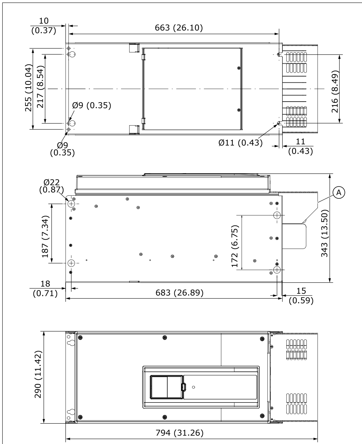
Fig. 3: Dimensions du convertisseur de fréquence, MR8, [mm (pouces)]
