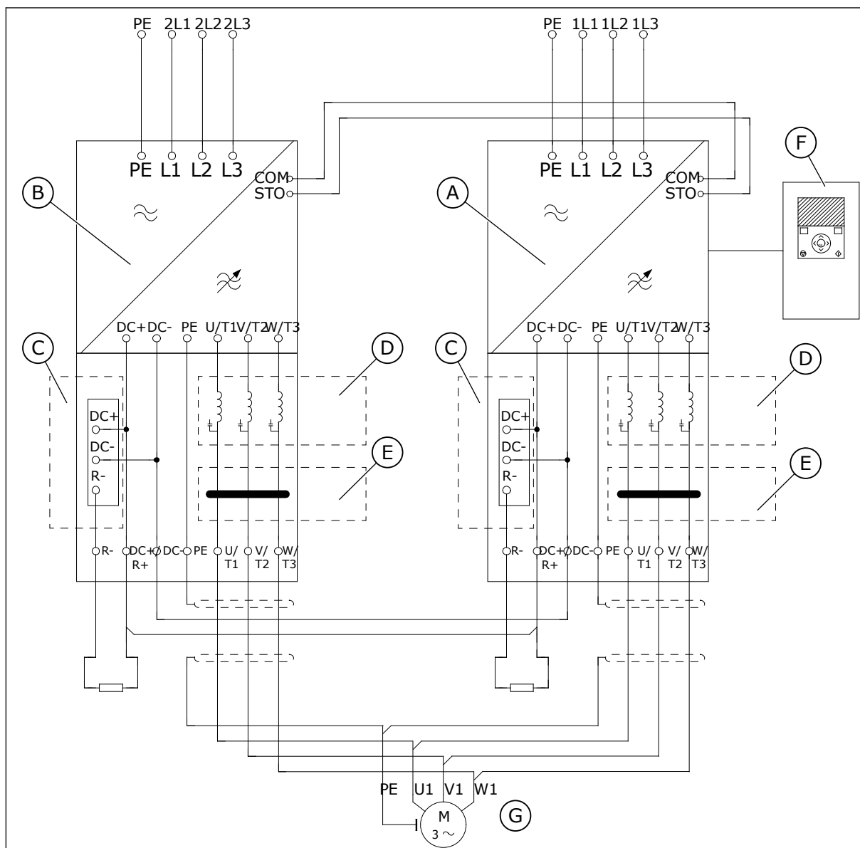
Fig. 12: Schéma général MR12 avec le module d'options
