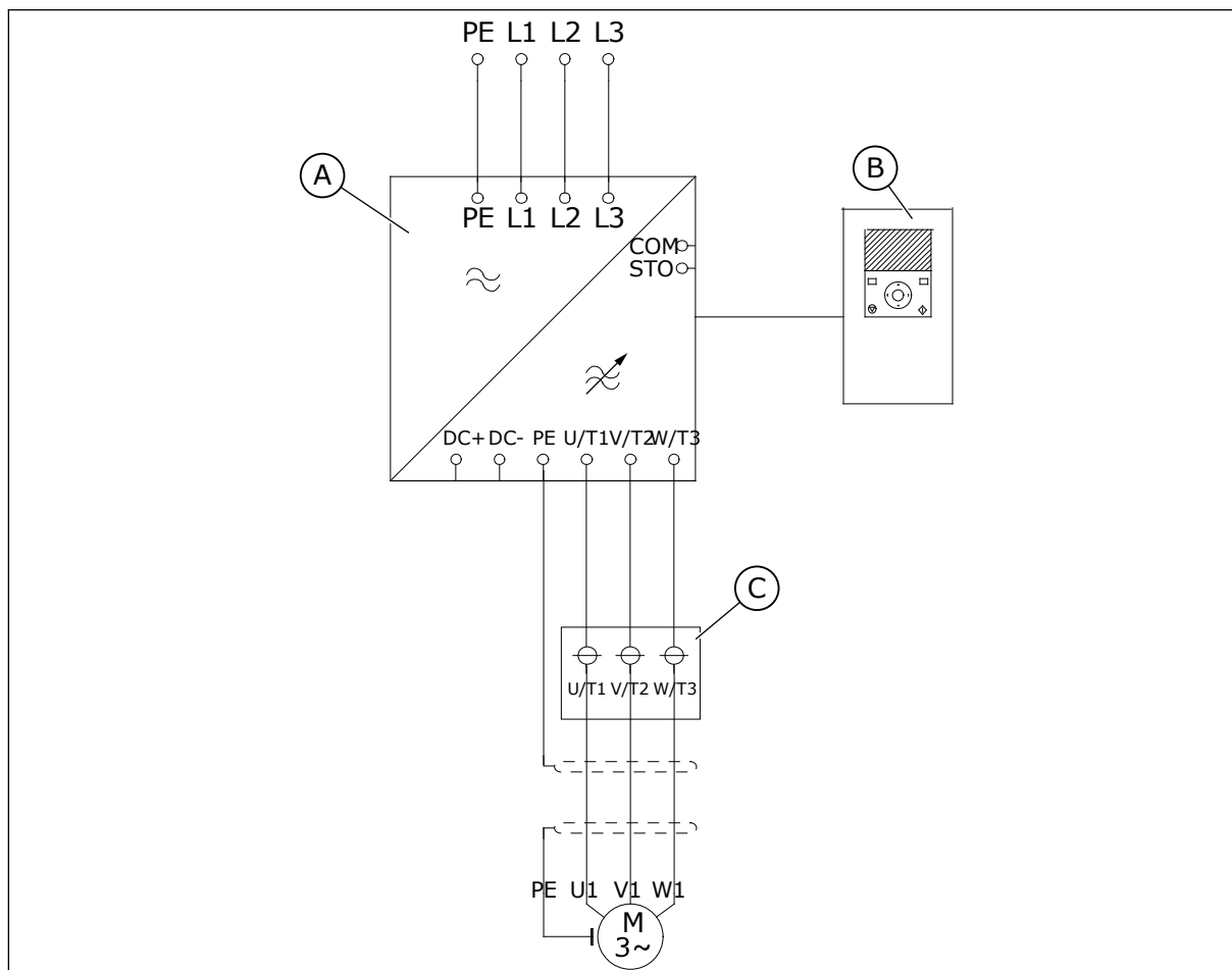
Fig. 9: Schéma général MR10 (sans les options)
