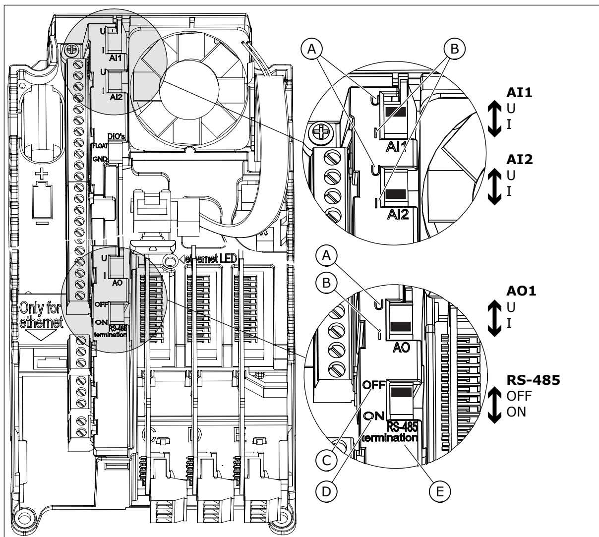
Fig. 22: Les sélections des interrupteurs DIP
