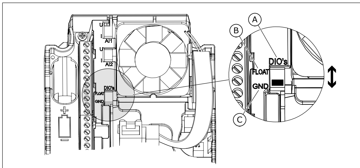
Fig. 23: Changez la position de cet interrupteur pour isoler les entrées logiques de la terre
