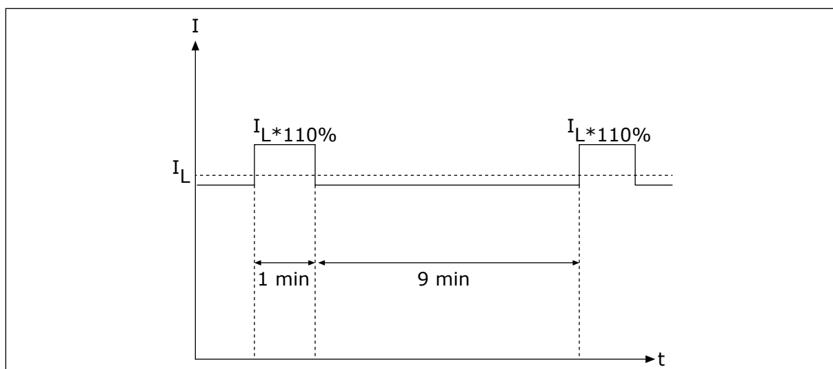
Fig. 30: Faible surcharge dans Vacon® 100 FLOW
