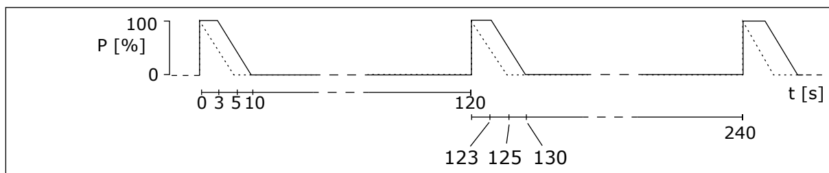
Fig. 29: Les cycles des impulsions de régime normal et de régime intensif
