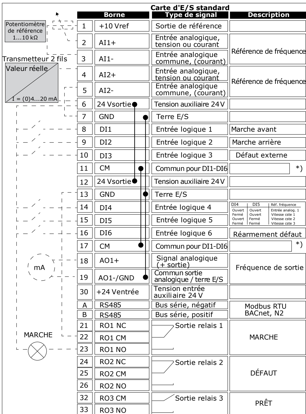
Fig. 19: Signaux des bornes de commande sur la carte d'E/S standard, et un exemple de connexion. Si vous incluez le code d'option +SBF4 dans votre commande, la sortie de relais 3 est remplacée par une entrée de thermistance.
