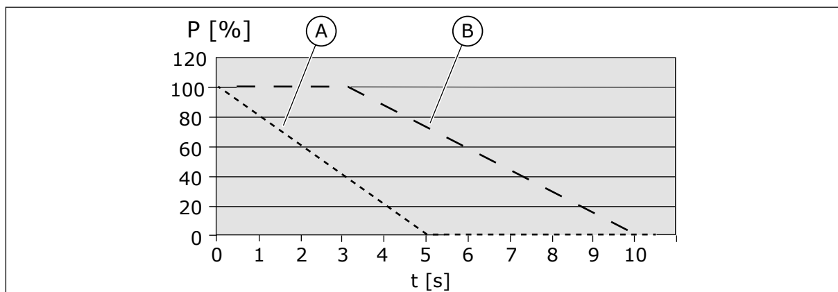
Fig. 28: Les impulsions de régime normal et de régime intensif
