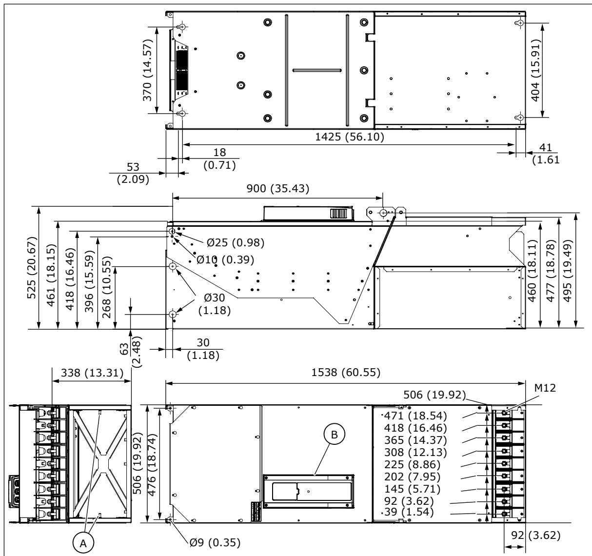
Fig. 7: Dimensions avec le module d'options [mm (pouces)]
