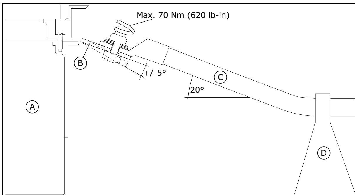
Fig. 17: Support mécanique pour les câbles lorsque le convertisseur n'a pas de module d'options
