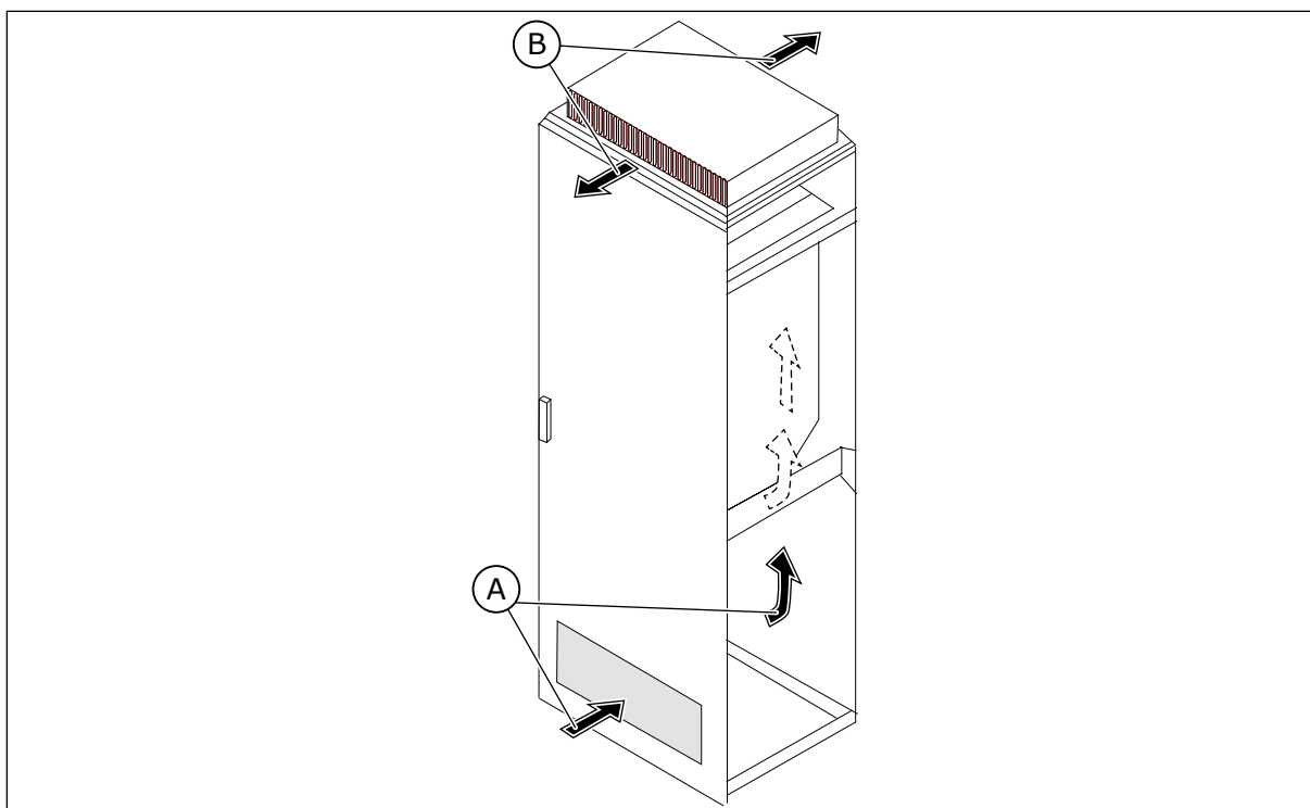
Fig. 15: L'air de refroidissement doit circuler librement dans l'armoire
