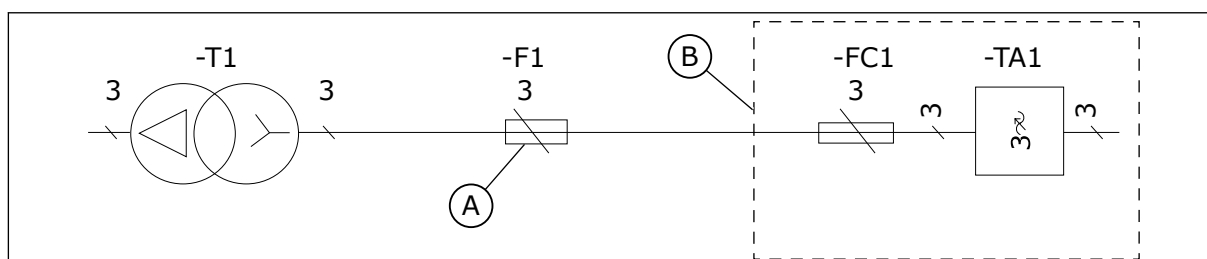
Fig. 16: Emplacement des fusibles
