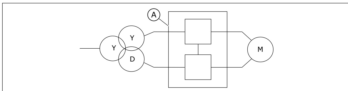
Fig. 13: Fonctionnement à 12 pulses de MR12
