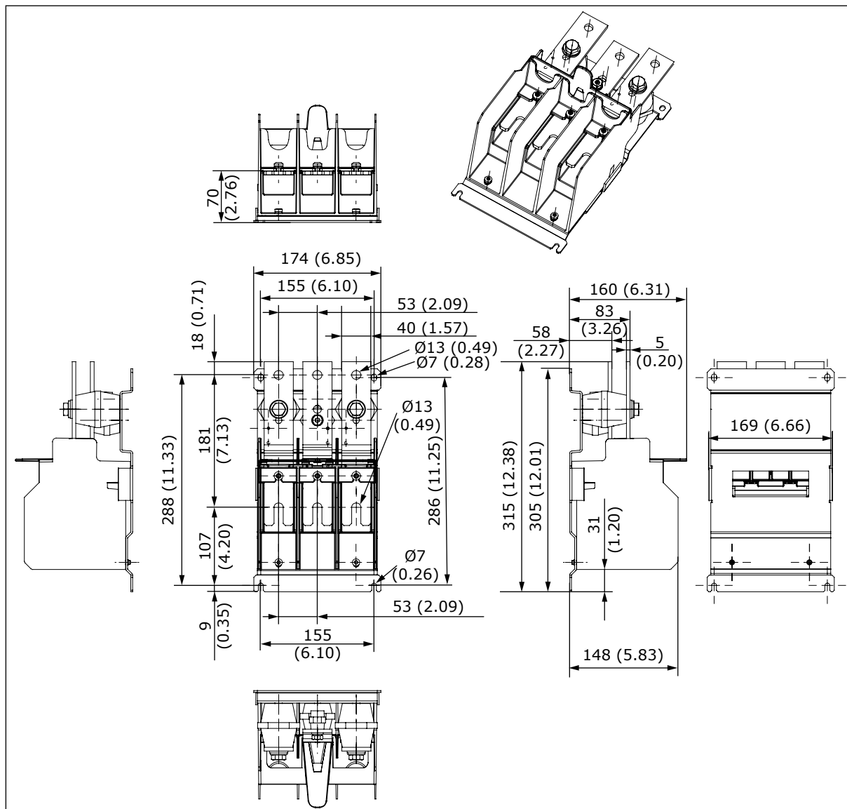
Fig. 6: Dimensions du bloc de raccordement de puissance externe optionnel (+PCTB), utilisé sans le module d'options [mm (pouces)]
