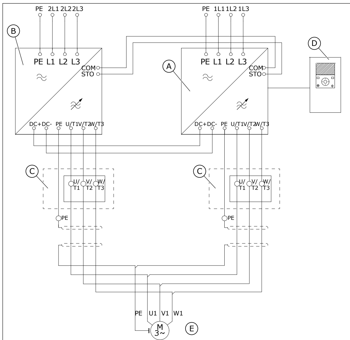
Fig. 11: Schéma général MR12 sans le module d'options
