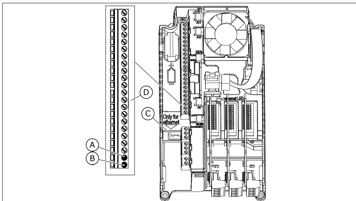
Fig. 24: Les connexions Ethernet et RS485
