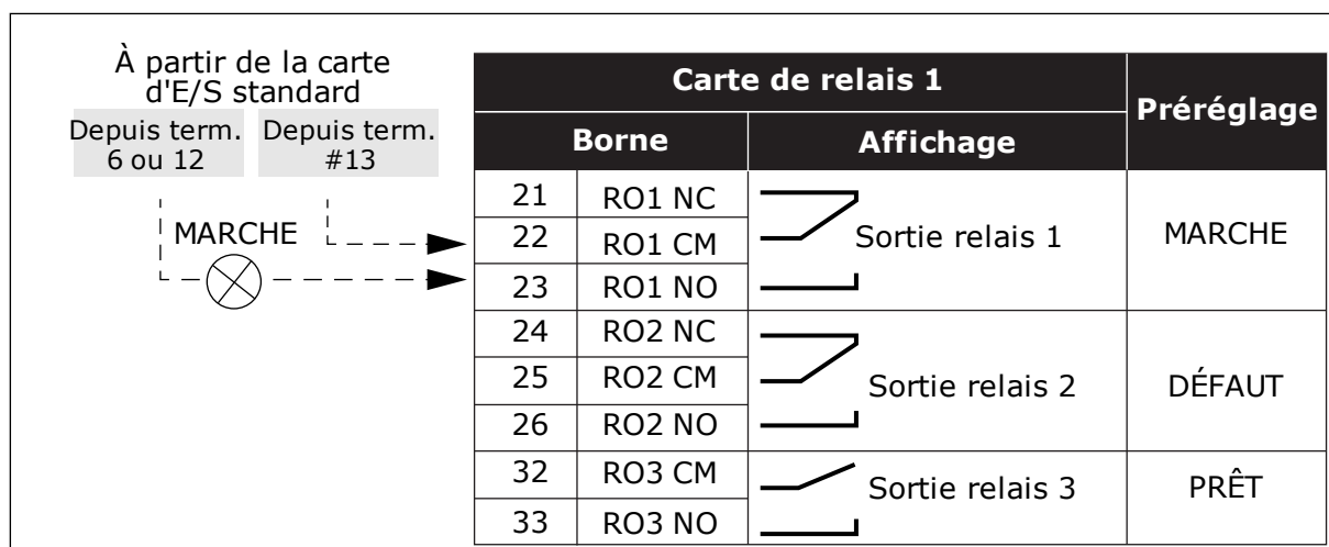
Fig. 20: La carte de relais standard (+SBF3)
