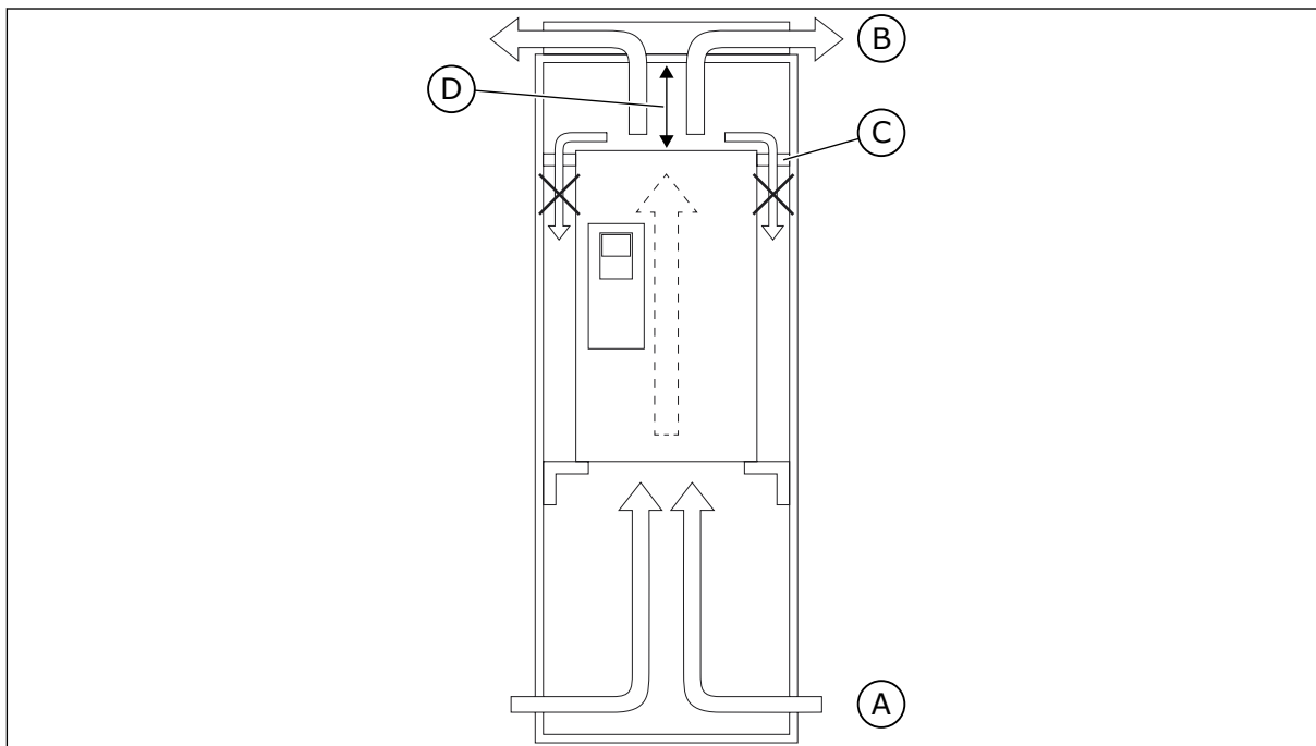
Fig. 14: Circulation correcte de l'air de refroidissement dans l'armoire
