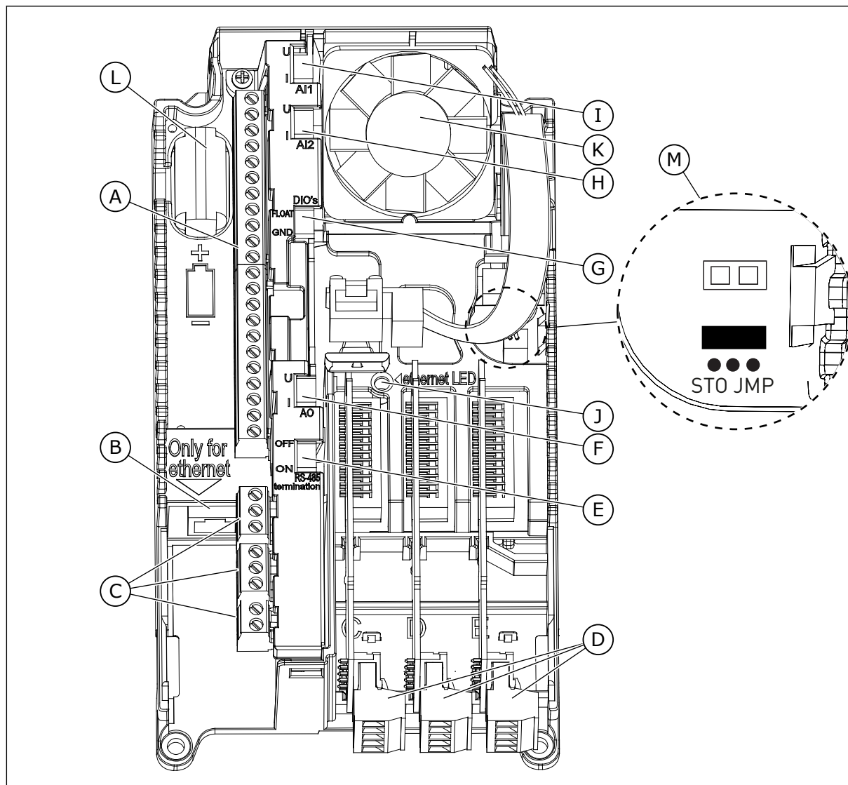
Fig. 18: Les composants de l'unité de commande
