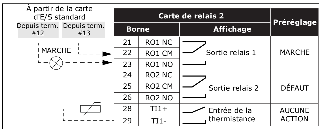
Fig. 21: La carte de relais optionnelle (+SBF4)
