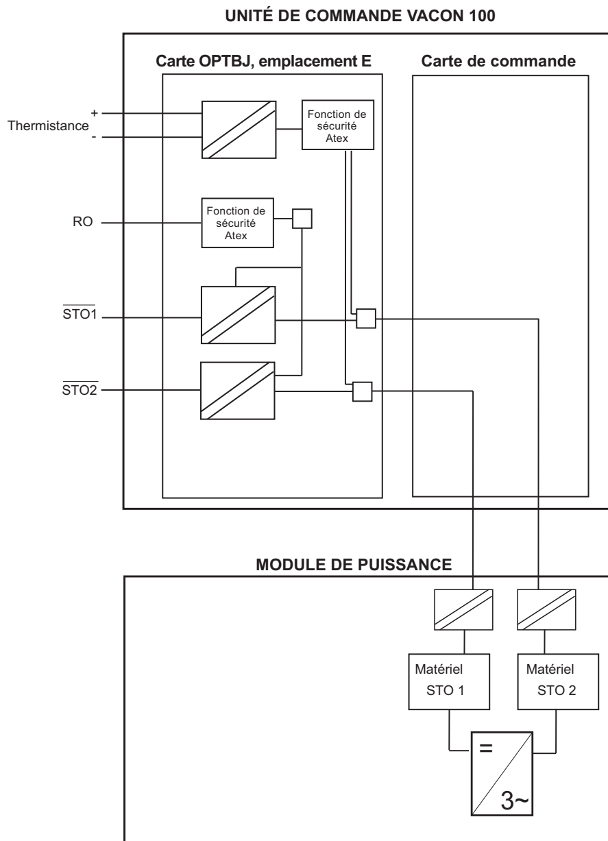
Figure 15. Principe de la fonction de thermistance dans le convertisseur de fréquence de la gamme VACON® 100 avec carte OPTBJ, MR4-10
