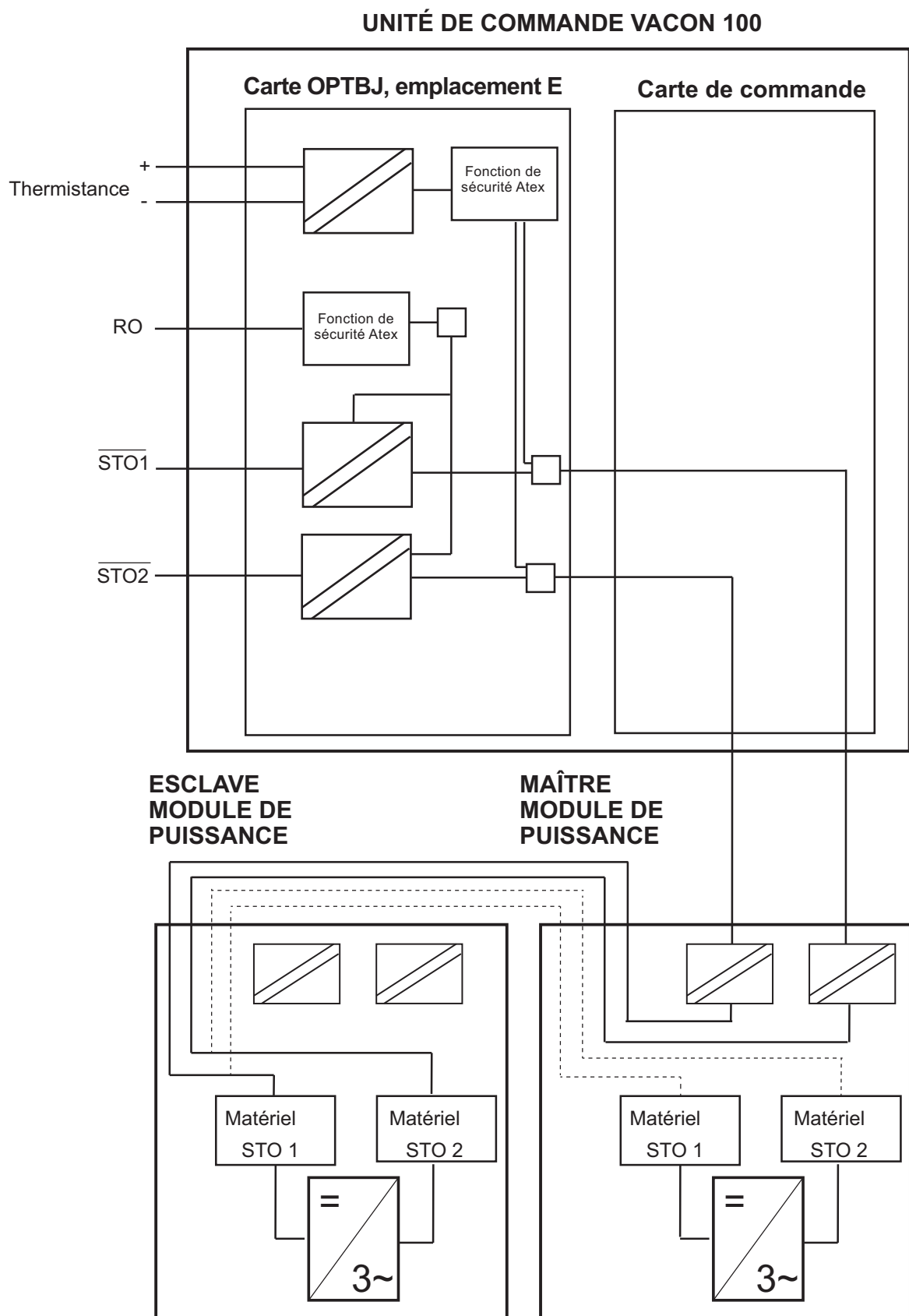
Figure 16. Principe de la fonction STO avec carte OPTBJ et carte de commande de la gamme VACON® 100 MR12
