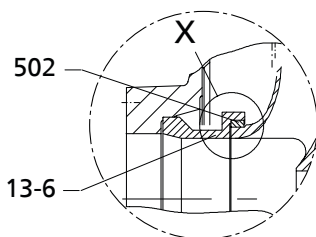
Fig. 15: K impeller
