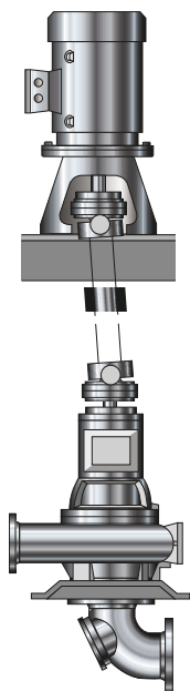
III. 9: Sewatec - vertical (VGW) : groupe motopompe avec plaque-support pour la pompe et le moteur, cadre-porteur, lanterne d'entraînement, coude d'aspiration et arbre articulé
