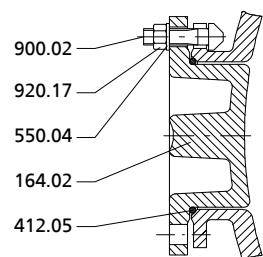
III. 25: Trou de visite, support de palier S01 à S08
