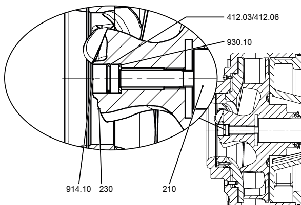
III. 24: Fixation de roue pour support de palier S07 (forme de roue D)
