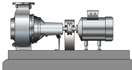
III. 5: Sewatec - 3E (3EN/3ENH) : groupe motopompe avec entraînement directement accouplé, socle, accouplement (avec ou sans entretoise), protège-accouplement et réglage en hauteur du moteur
