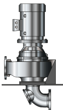
III. 10: Sewabloc - vertical (V) : groupe motopompe avec moteur directement raccordé par bride (forme de construction B5/V1), avec plaque-support et coude d'aspiration, installation souterraine
