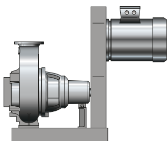
III. 2: Sewatec - 3H (3HZ) : groupe motopompe avec socle, entraînement poulie-courroie et protège-courroie
