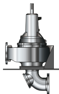
III. 7: Sewatec - vertical (V) : pompe à arbre nu, plaque-support et coude d'aspiration
