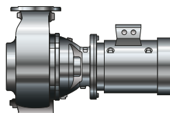
III. 6: Sewabloc : groupe motopompe avec moteur directement raccordé par bride (forme de construction B5/V1)
