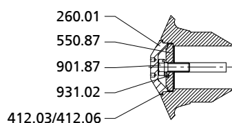
III. 23: Fixation de la roue pour support de palier S07 et S08 (forme de roue E et K) sauf taille Sewatec 500-632
