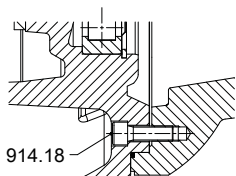
III. 16: Détail X
