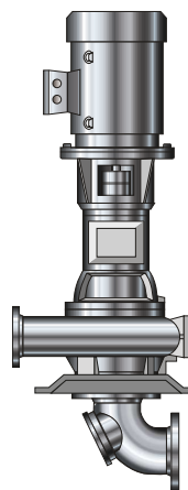
III. 8: Sewatec - vertical (VU) : groupe motopompe avec plaque-support, lanterne d'entraînement, accouplement, protège-accouplement et coude d'aspiration
