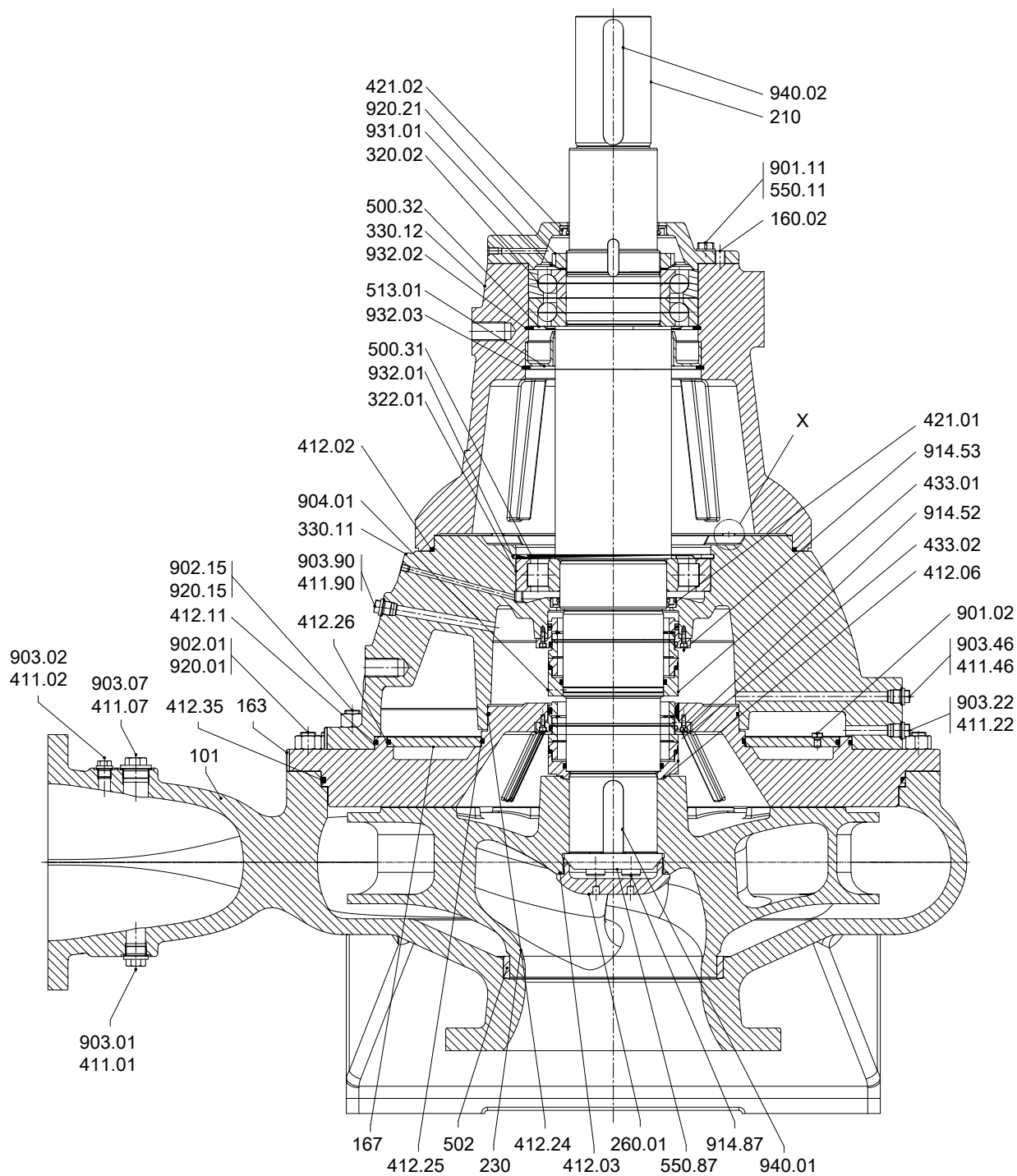
III. 15: Sewatec avec support de palier S09, S10
