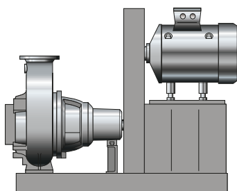
III. 3: Sewatec - 3H (3HM) : groupe motopompe avec socle, entraînement poulie-courroie, protège-courroie et support de moteur
