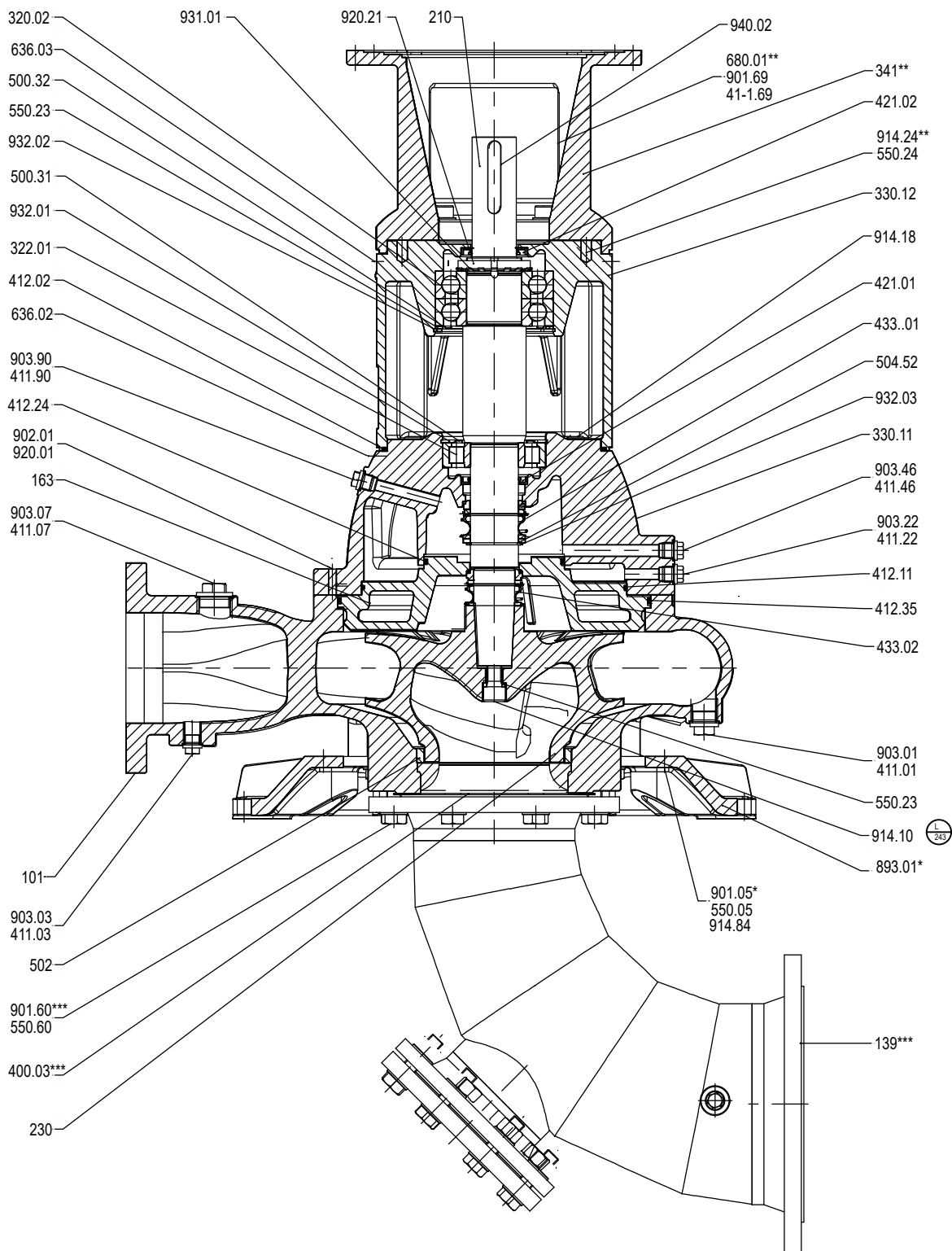
III. 14: Sewatec avec roue E - pompe pour installation souterraine, version à arbre articulé
