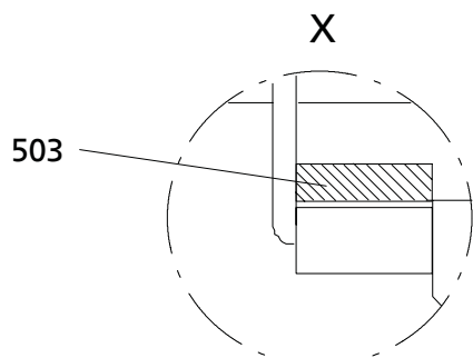
III. 20: Détail X : bague d'usure de la roue pour roue K
