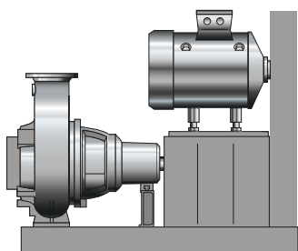
III. 4: Sewatec - 3H avec réducteur (3HVG) : groupe motopompe avec socle, accouplement (avec ou sans entretoise), protège-accouplement, support de réducteur, réducteur, support de moteur, entraînement poulie-courroie et protège-courroie
