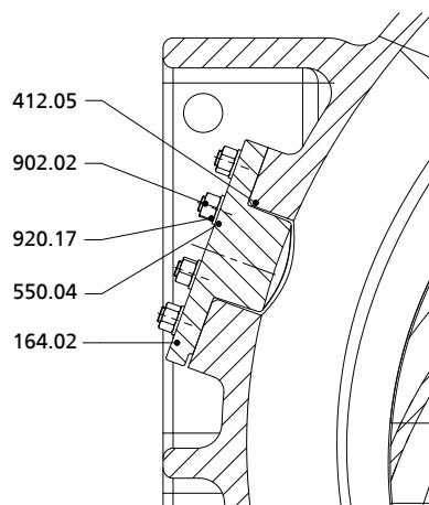
III. 26: Trou de visite, support de palier S09 et S10
