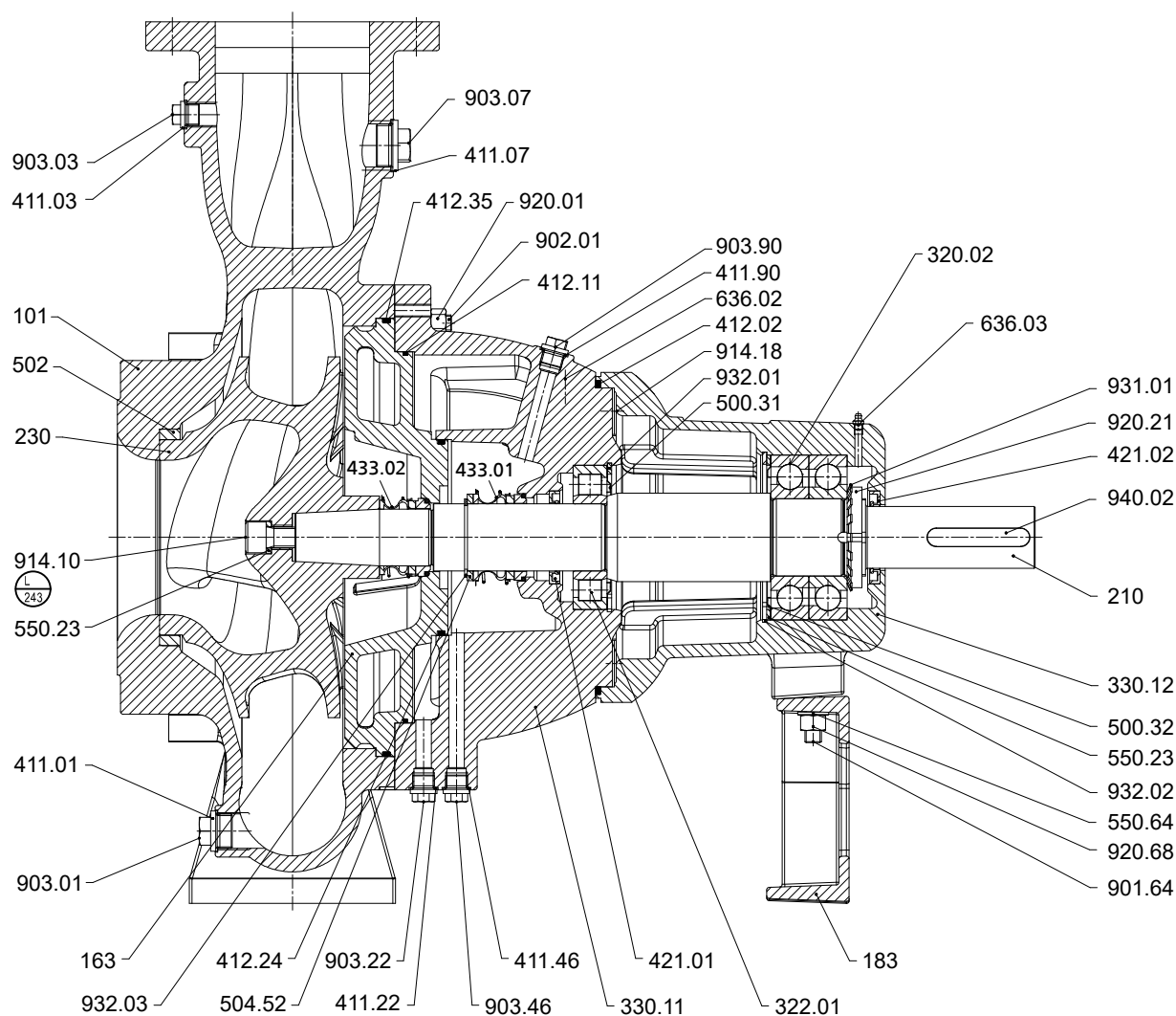
III. 13: Sewatec avec support de palier S05 à S08
