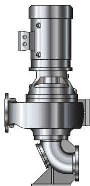
III. 11: Sewabloc - vertical (VF) : groupe motopompe avec moteur directement raccordé par bride (forme de construction B5/V1), avec pied d'assise d'aspiration
