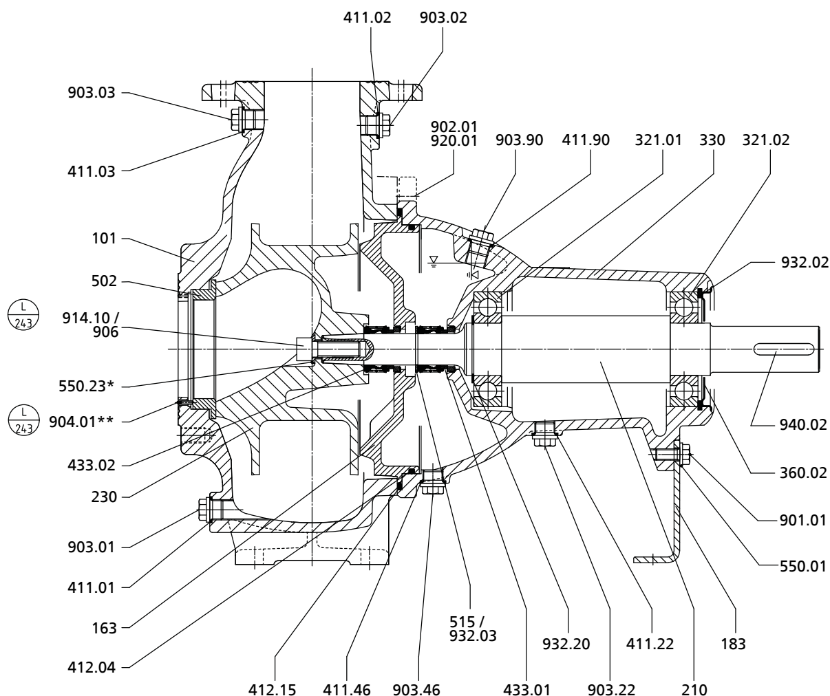
III. 12: Plan d'ensemble Sewatec - Support de palier S01, S02, S03, S04 avec forme de roue E; * si prévu, ** uniquement pour tailles E 100-250, E 100-253, E 100-317, E 150-317, K 100-253, K 100-254, K 100-316
