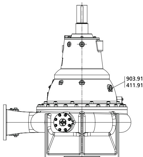
III. 27: Trou auxiliaire lié à la fabrication, supports de palier S09 et S10
