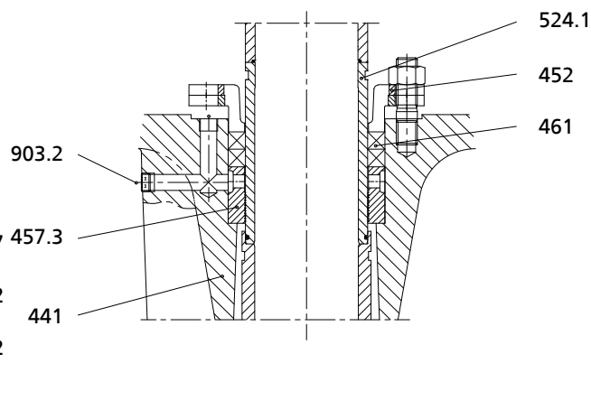
Plan de détail : garniture de presse-étoupe \geq 7 bar [99,5 psi] de pression de refoulement
