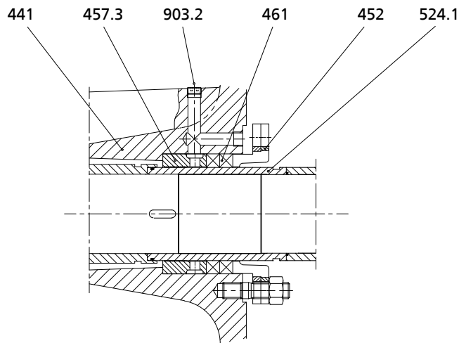
III. 7: Installation horizontale : * = uniquement pour version avec garniture de presse-étoupe < 7 bar [99,5 psi] de pression de refoulement
