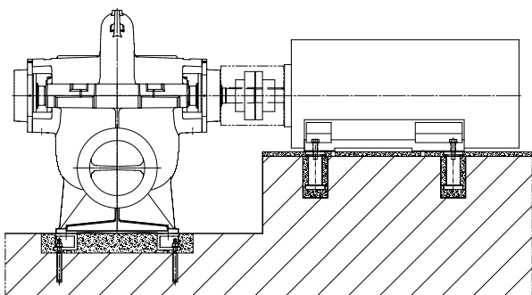
III. 2: 2E : pompe et moteur sur rails de fondation
