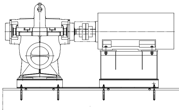
III. 4: 4E : pompe et moteur installés sur des châssis séparés
