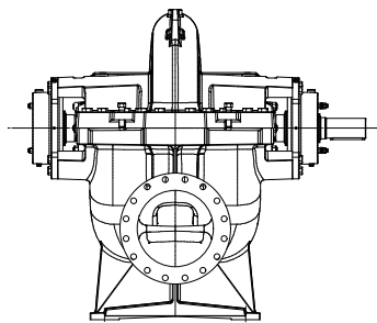
III. 1: Fig. 0 : Pompe à arbre nu
