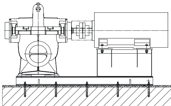
III. 3: 3E : pompe et moteur montés sur châssis commun
