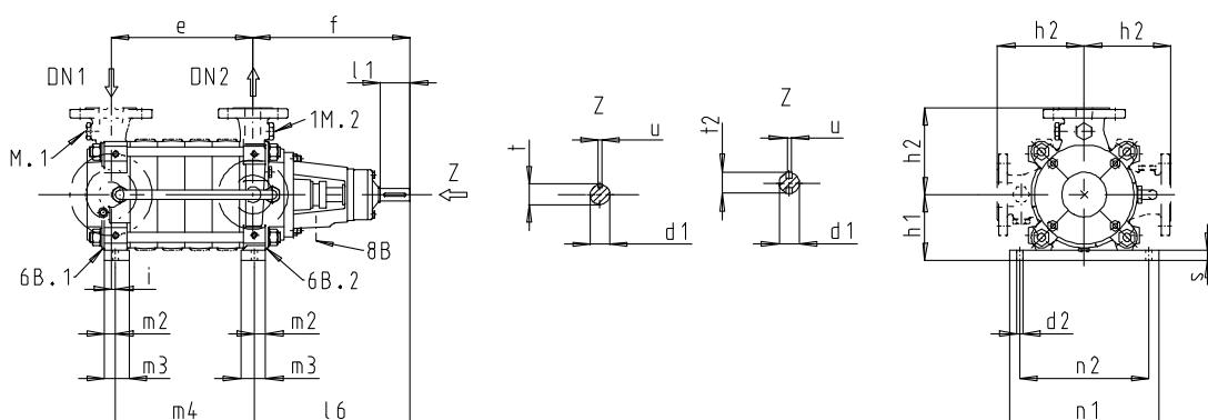
Fig. 2: Multitec B dimensions 36)
