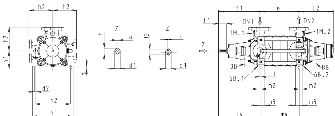
Fig. 4: Multitec D dimensions 36)
