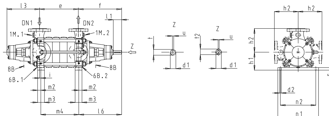
Fig. 3: Multitec C dimensions 36)
