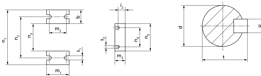
III. 2: Dimensions bout d'arbre et pieds de pompe
