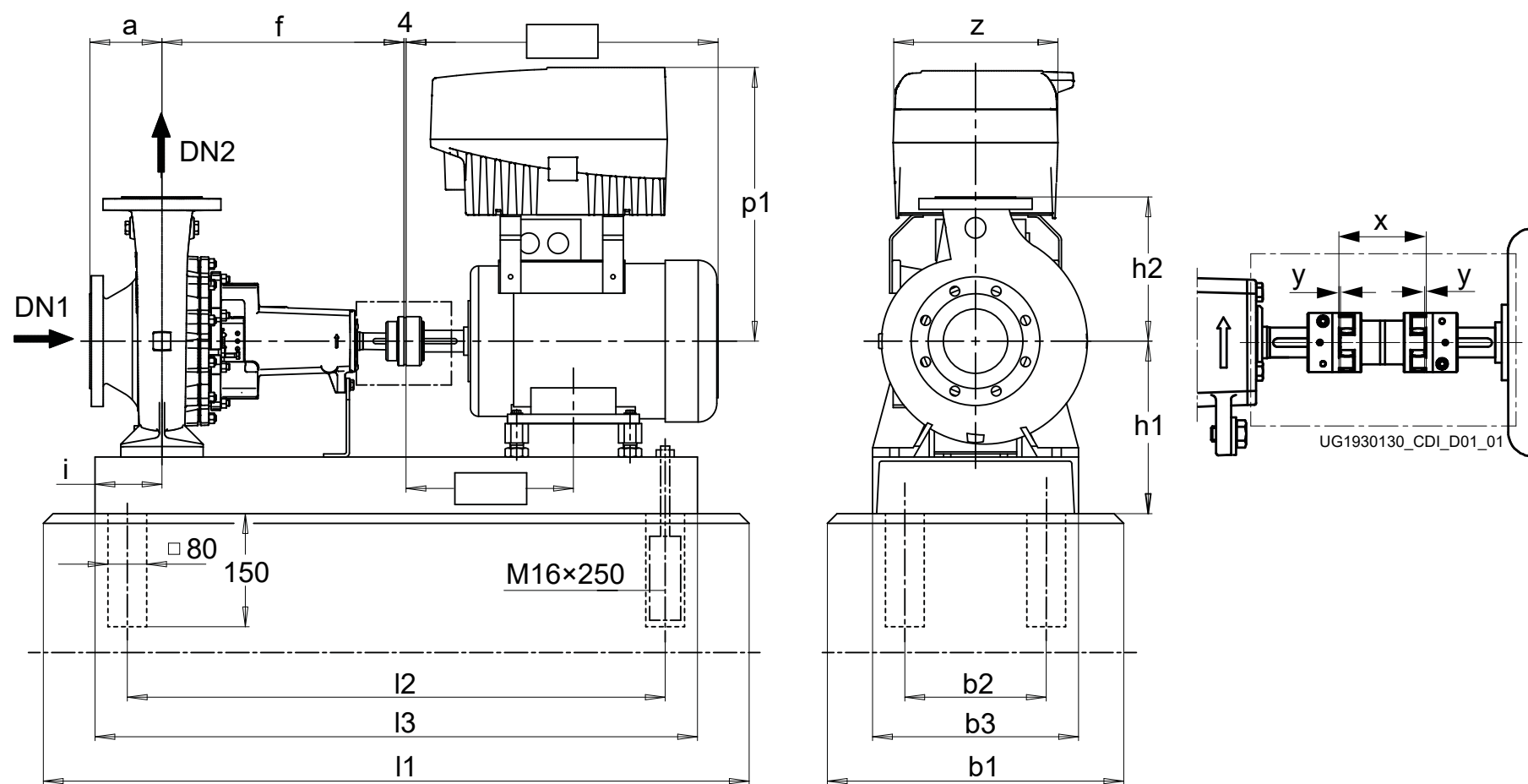
III. 5: Dimensions groupe motopompe avec accouplement (illustration A)
