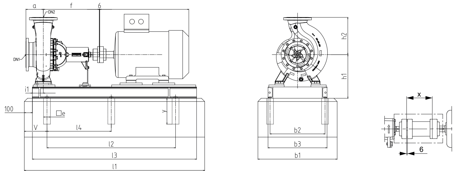
III. 7: Dimensions groupe motopompe avec accouplement
