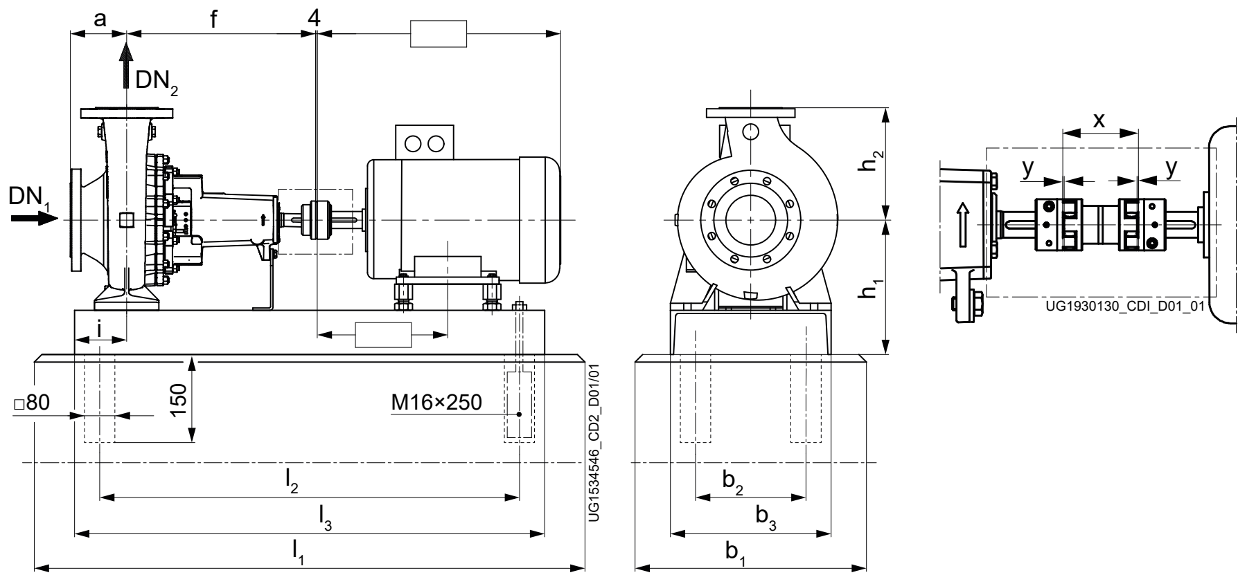
III. 3: Dimensions groupe motopompe avec accouplement (illustration A)
