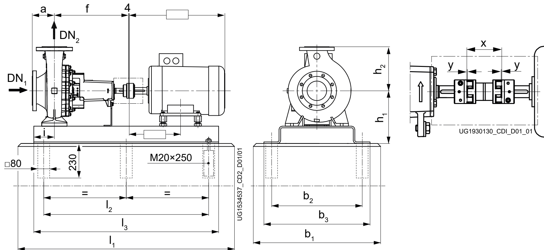
III. 4: Dimensions groupe motopompe avec accouplement à entretoise (illustration B)
