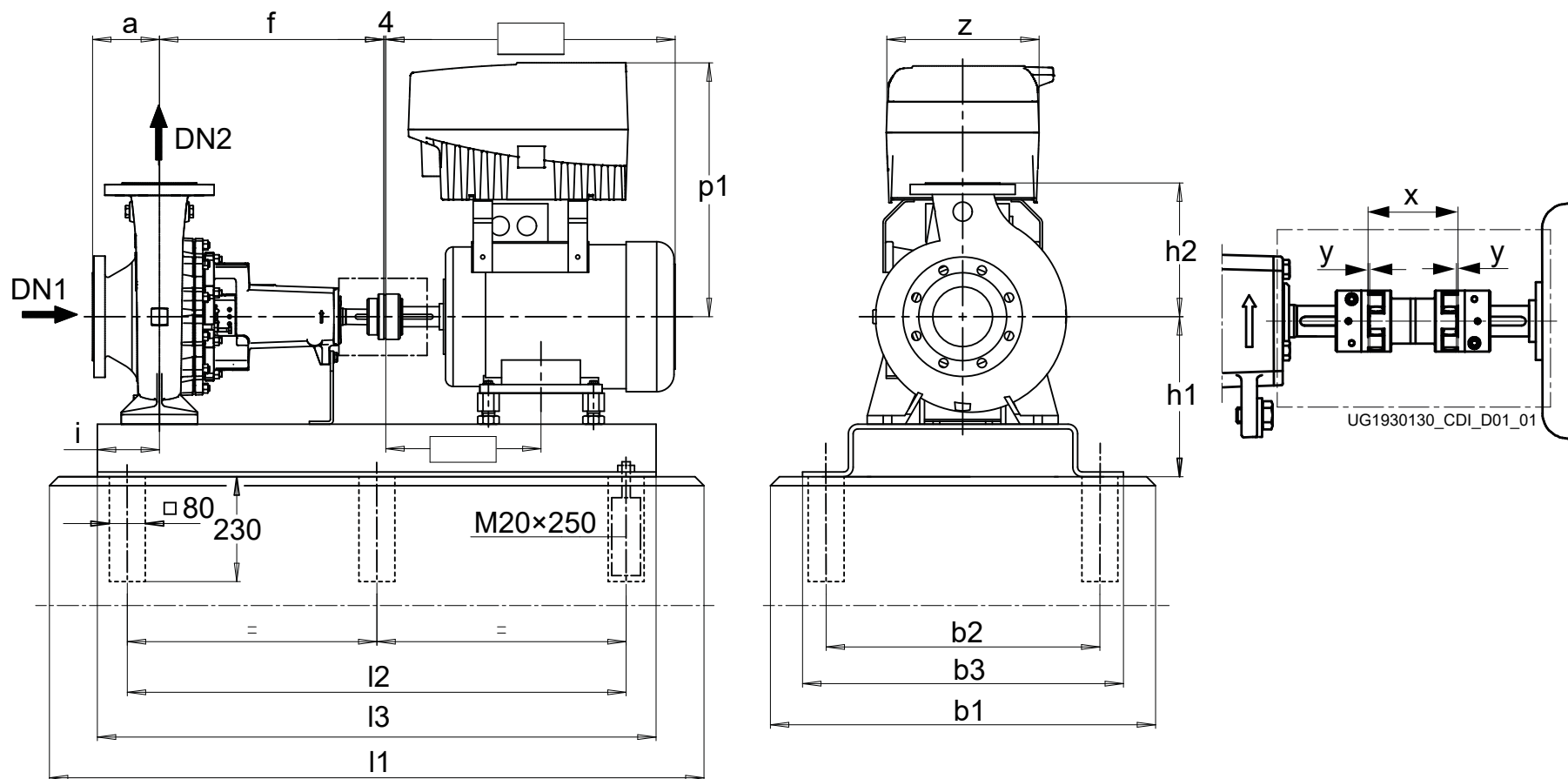
III. 6: Dimensions groupe motopompe avec accouplement à entretoise (illustration B)
