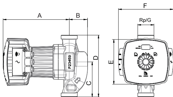
III. 4: Groupe motopompe à orifices filetés
