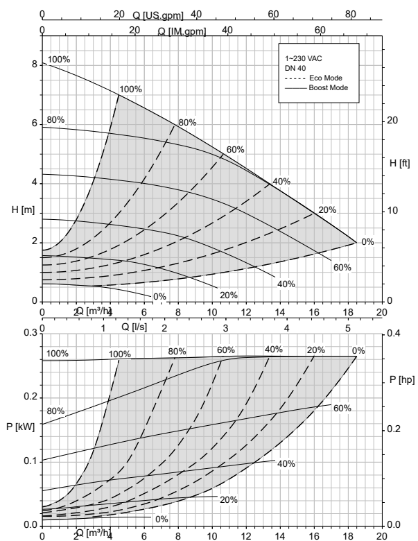
Calio 40-80 fonct. boucle ouverte, Eco-Mode
