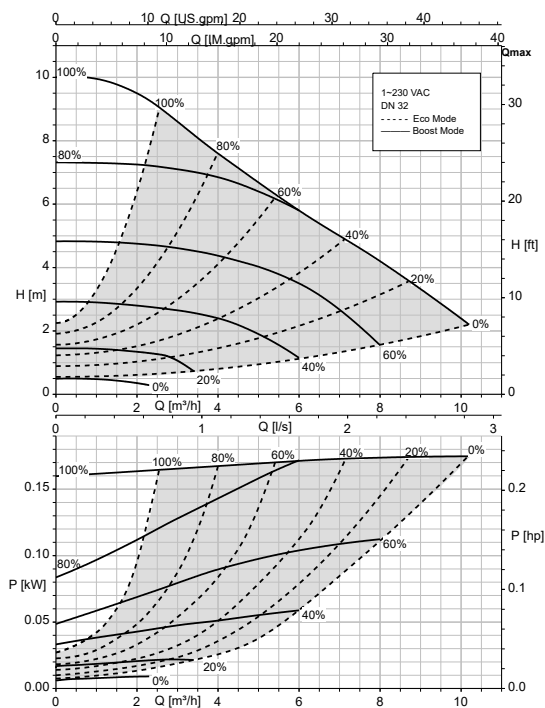
Calio 32-100 fonct. boucle ouverte, Eco-Mode
