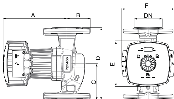
III. 5: Groupe motopompe à brides
