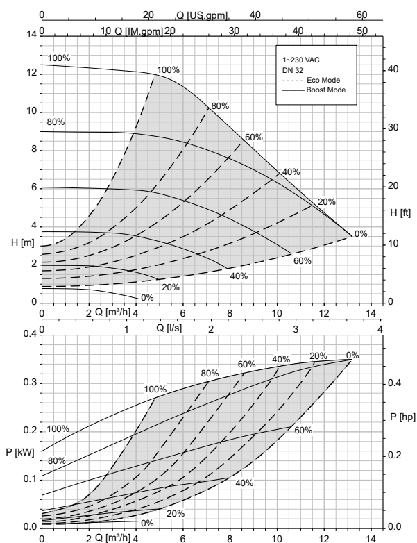
Calio 32-120 fonct. boucle ouverte, Eco-Mode
