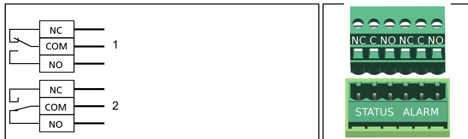
III. 11: Schéma de connexion report centralisé de défaut
