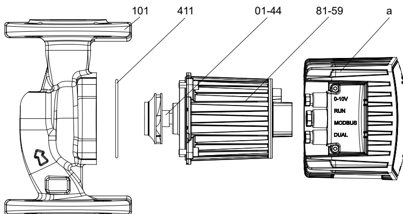
III. 30: Vue éclatée
