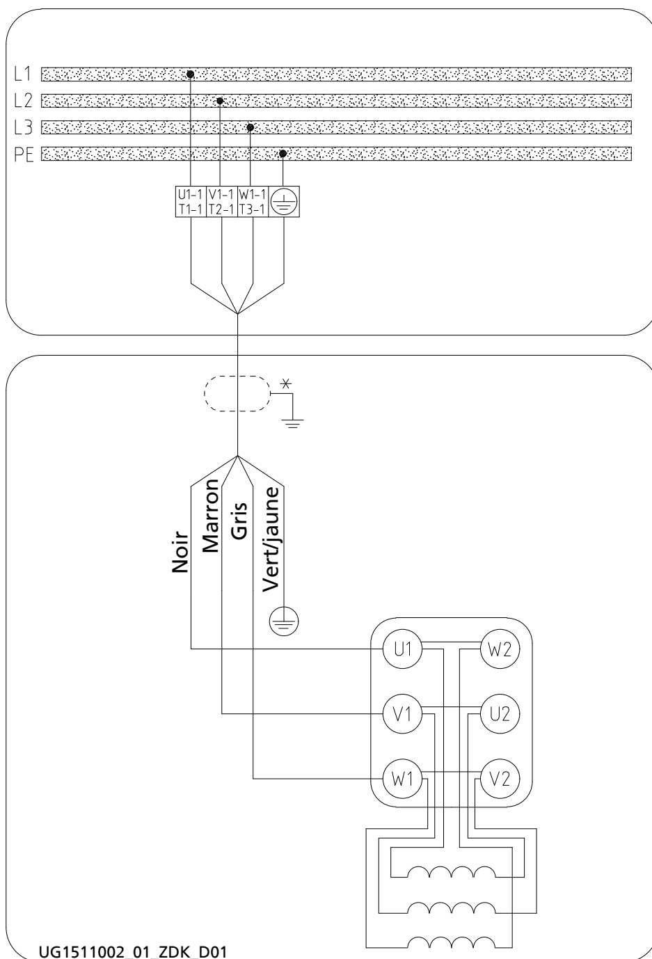
III. 50: Schéma électrique * câble blindé en option
