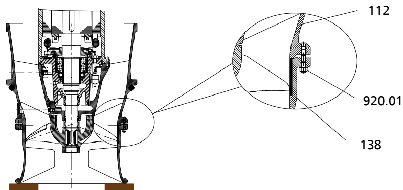
III. 32: Démontage de la tulipe d'entrée
