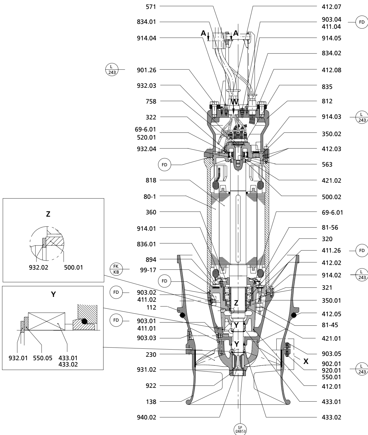
III. 47: Plan d'ensemble
