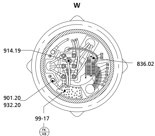
Détail W : vue du compartiment électrique
