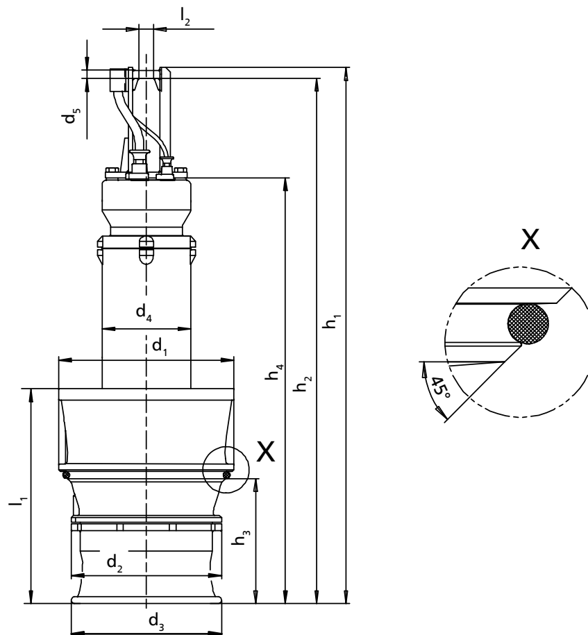
III. 54: Dimensions groupe motopompe
