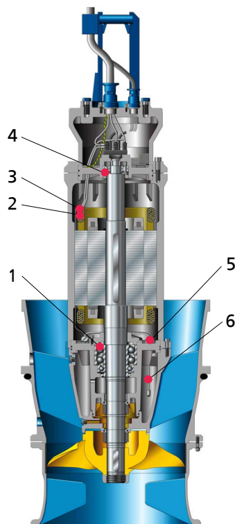
III. 25: Positions des capteurs
