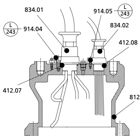
III. 38: Montage du passage de câble
