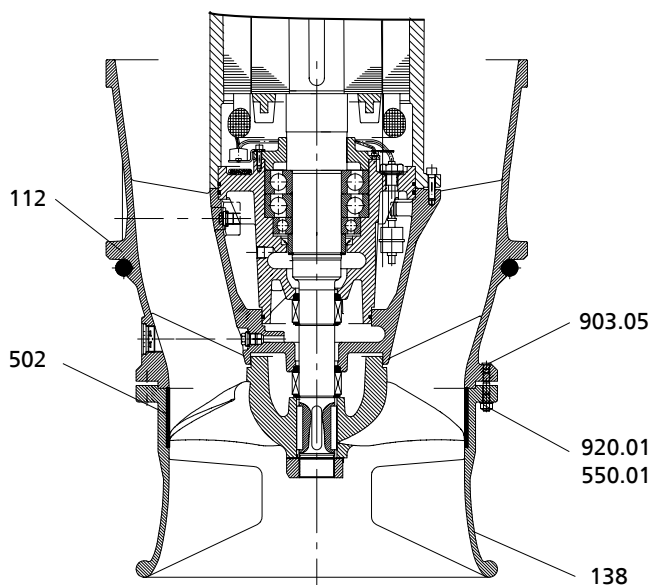
Détail X : vue de la bague d'usure, classe de pression A
