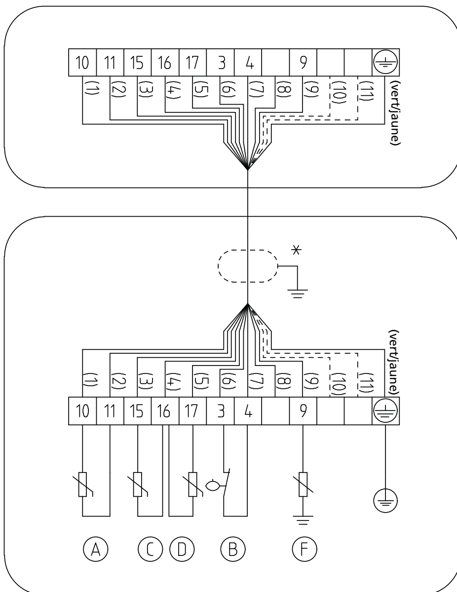
III. 51: Schéma de connexion capteurs pour groupes motopompes standard
