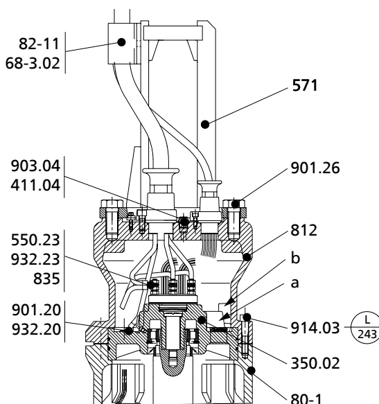
III. 39: Montage du fond de carcasse de moteur
