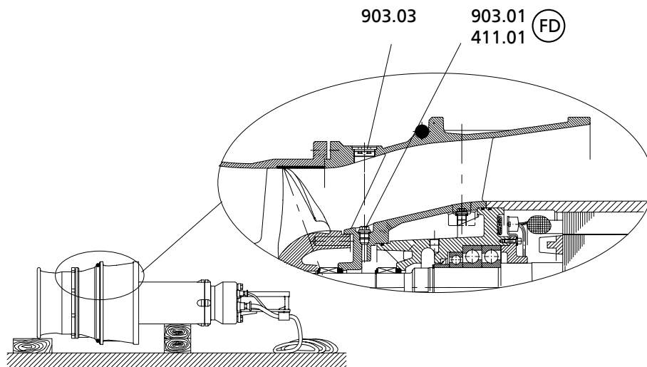
III. 31: Remplissage du lubrifiant liquide
