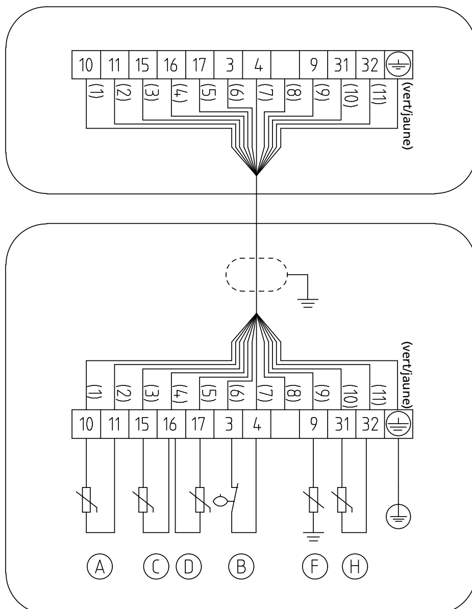
III. 52: Schéma de connexion pour groupe motopompe avec surveillance supplémentaire de la température du moteur par Pt100
