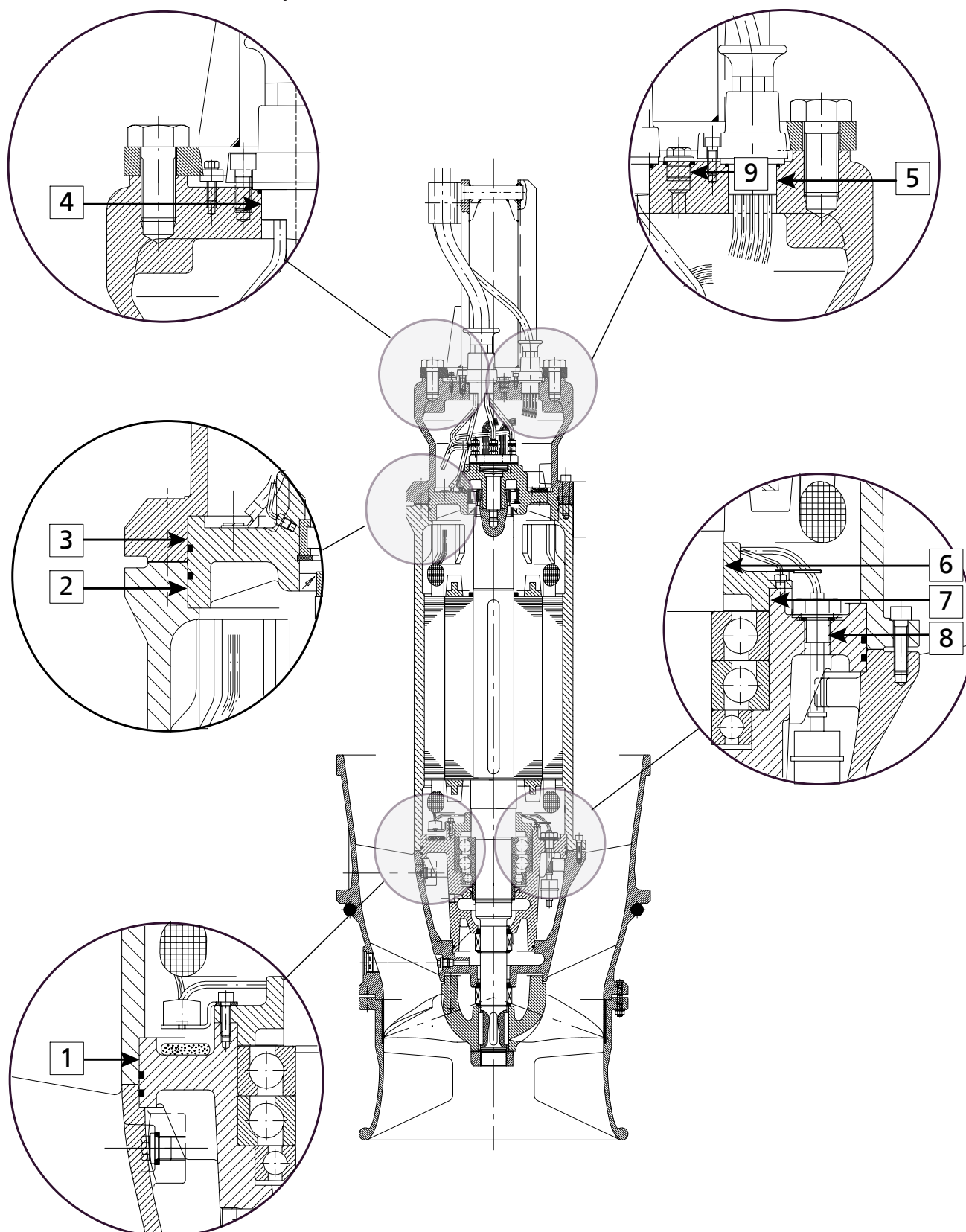
III. 53: Joints antidéflagrants
