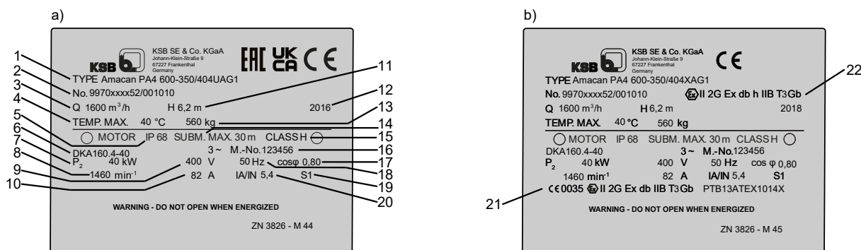
III. 5: Plaque signalétique (exemple) a) Groupe motopompe standard b) Groupe motopompe protégé contre les explosions
