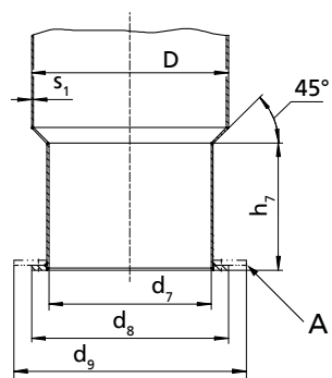
III. 55: Dimensions du tube
