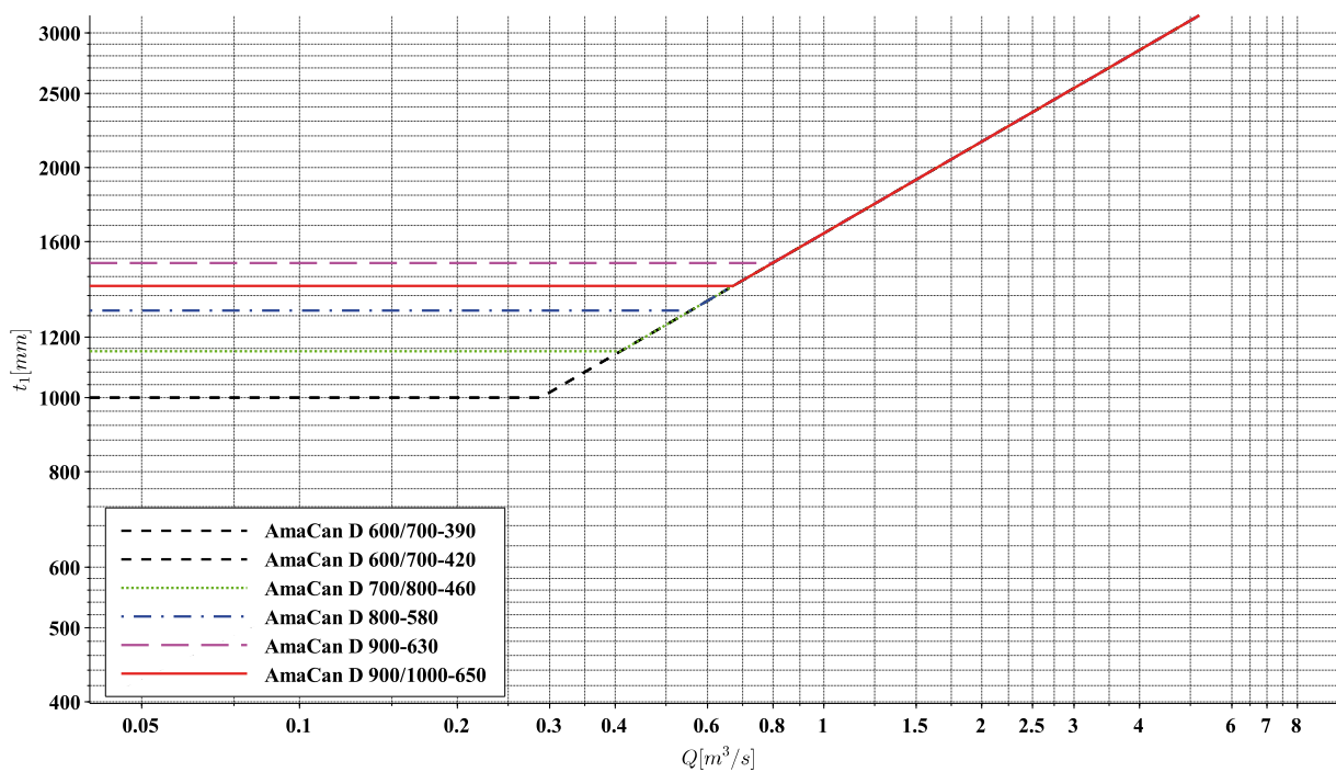
III. 5: Mode d'installation CUS : chambre ouverte, version avec plaque d'aspiration \varnothing d_9
