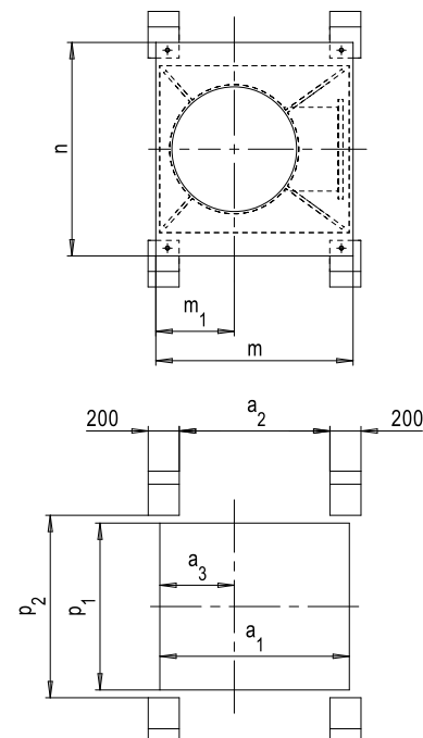
Détail X : plan de pose du tube, réserves de génie civil 23) Dimensions en [mm]
