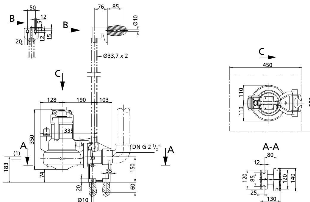
III. 24: Dimensions installation noyée stationnaire, pied d'assise droit G 2 ½", guidage par 1 barre
