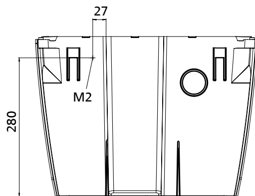
III. 3: Réalisation du perçage M2 [mm]
