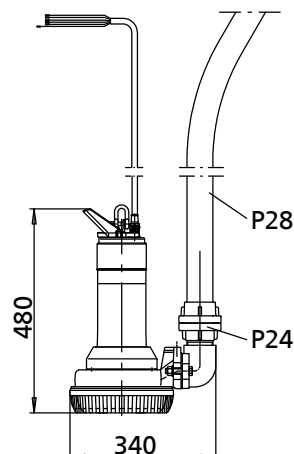
III. 11: AmaDrainer 5, installation transportable, passage libre 11 mm, sans interrupteur à flotteur, moteur triphasé, sans enveloppe de refroidissement
