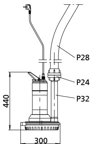
III. 9: AmaDrainer 4, installation transportable, passage libre 10 mm, sans interrupteur à flotteur, moteur monophasé, sans enveloppe de refroidissement
