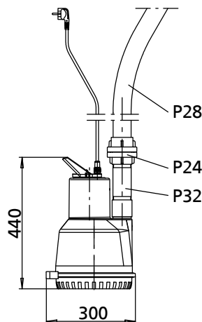
III. 10: AmaDrainer 5, installation transportable, passage libre 10 mm, sans interrupteur à flotteur, moteur monophasé, avec enveloppe de refroidissement
