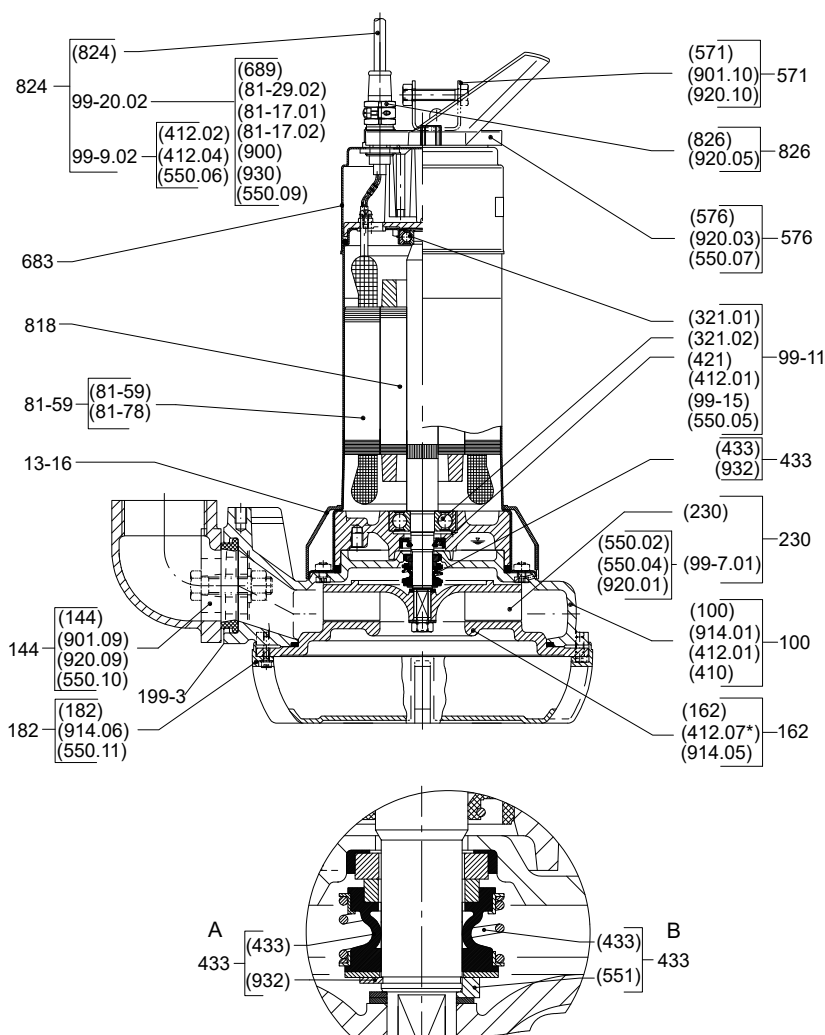
III. 16: Plan d'ensemble AmaDrainer 522 SD/11
