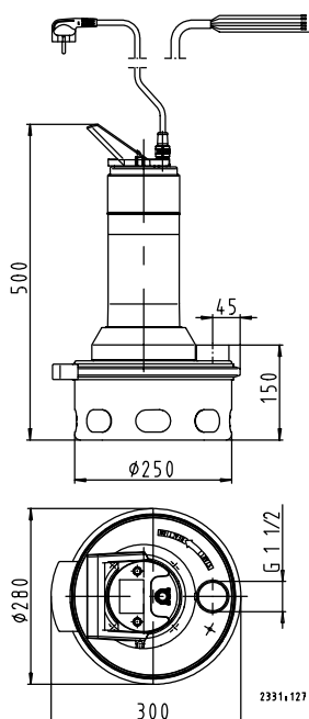
III. 2: AmaDrainer 4, passage libre 35 mm, sans enveloppe de refroidissement
