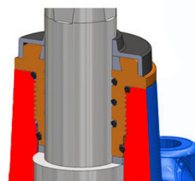
Étanchéité haut de vanne
