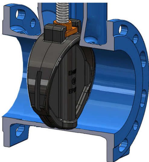
Étanchéité amont/aval
