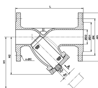
DN50-80
