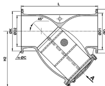
DN350-400
