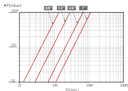
Diagramme de perte de charge
