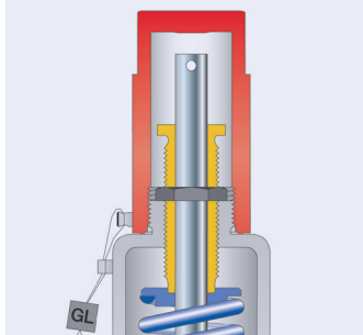
Test gag J69: H4 J70: H2 K05: H1 K27: H6
