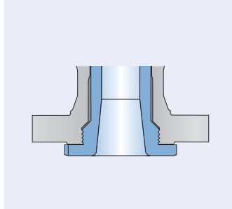
Flange drillings acc. to DIN EN 1092-1
