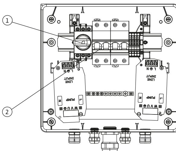
Fig. 2: Coffret d'alimentation réseau
