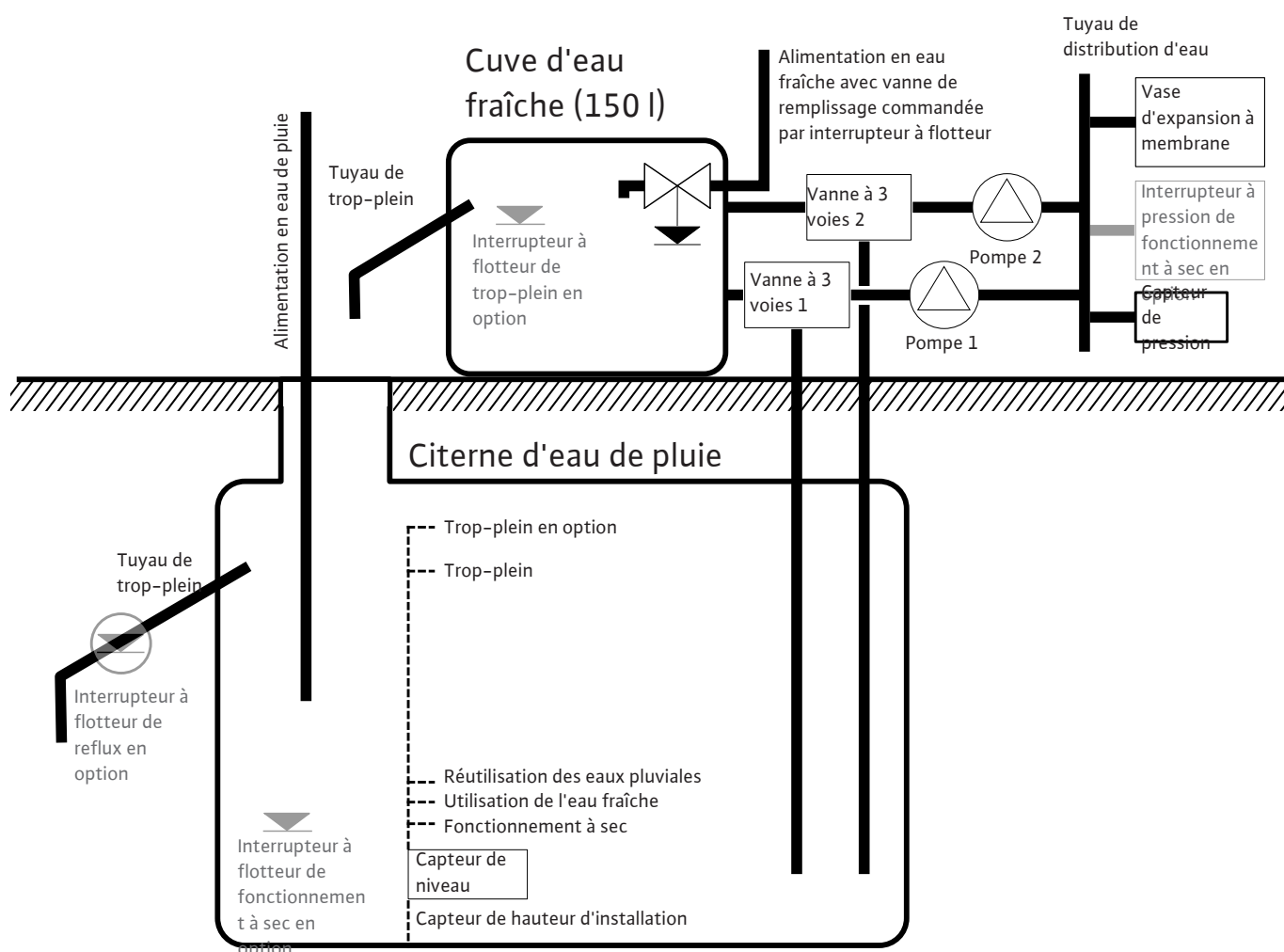
Fig. 20: Représentation schématique du principe de fonctionnement de l'AF150
