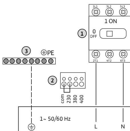
Fig. 3: Alimentation réseau Control EC-rF
