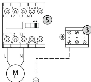
Fig. 4: Raccordement de la pompe
