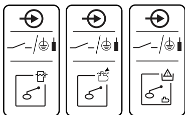
Fig. 10: Symbole dans l'aperçu du raccordement
