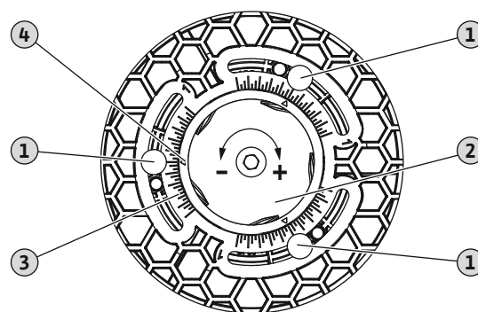
Fig. 8: Réglage de l'écartement de roue (crépine d'aspiration démontée)
