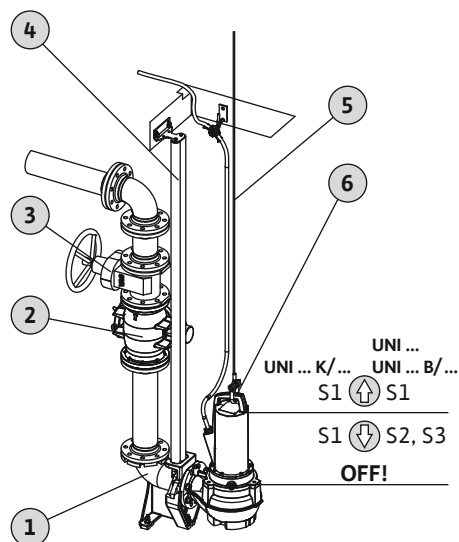
Fig. 5: Installation immergée stationnaire
