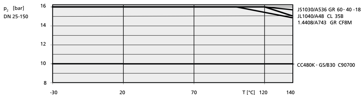
III. 1: Limites des pressions de pompe et des températures DN 25 - DN 150 pour ETN 26)
