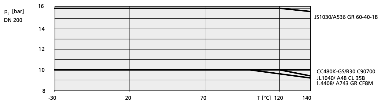
III. 2: Limites des pressions de pompe et des températures DN 200 pour ETN 26)
