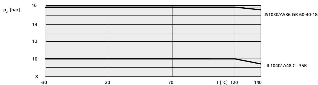
III. 3: Limites des pressions de pompe et des températures 27) ETNE 25)
