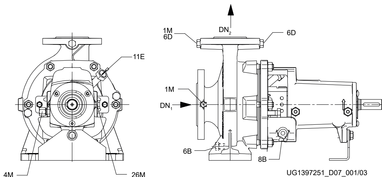
III. 7: Version avec lubrification à la graisse
