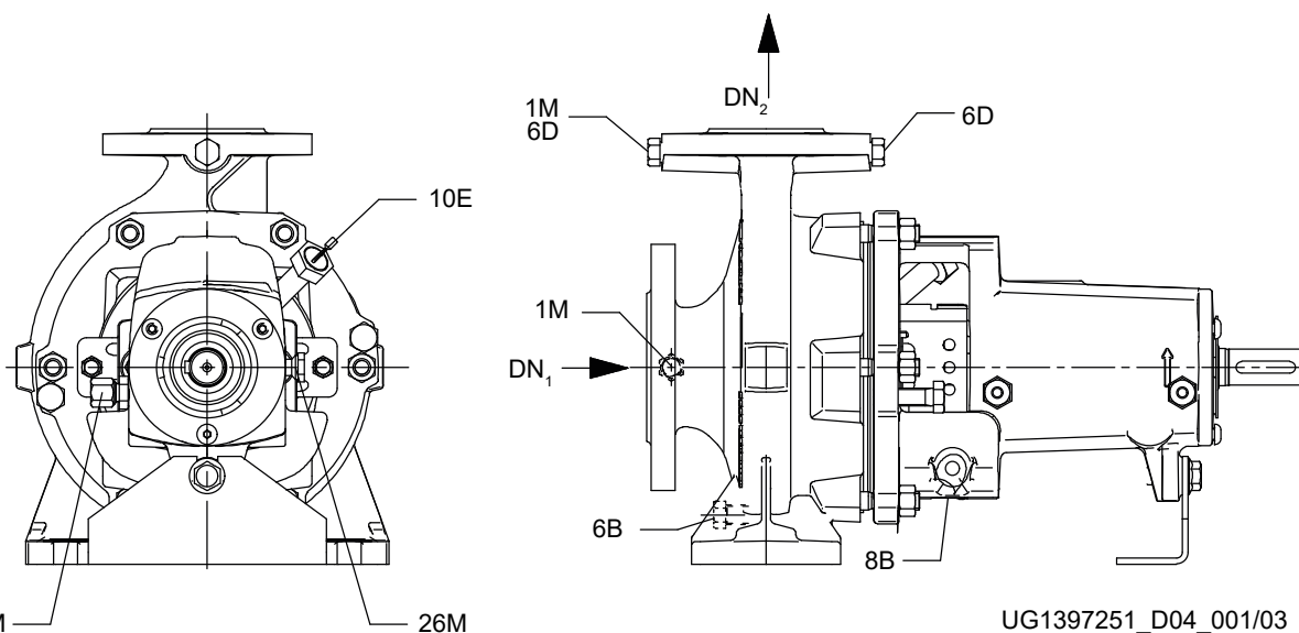
III. 8: Version avec lubrification à la graisse
