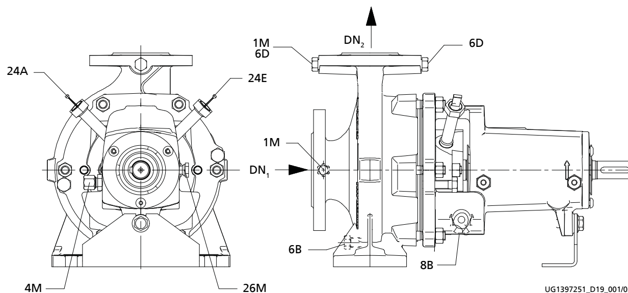
III. 9: Version avec lubrification à la graisse
