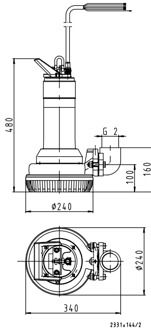
III. 4: AmaDrainer 5, passage libre 11 mm, sans enveloppe de refroidissement
