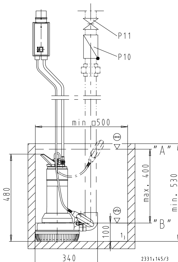
III. 8: AmaDrainer 5, pompe simple, passage libre 11 mm, avec interrupteur à flotteur, moteur triphasé, sans enveloppe de refroidissement
