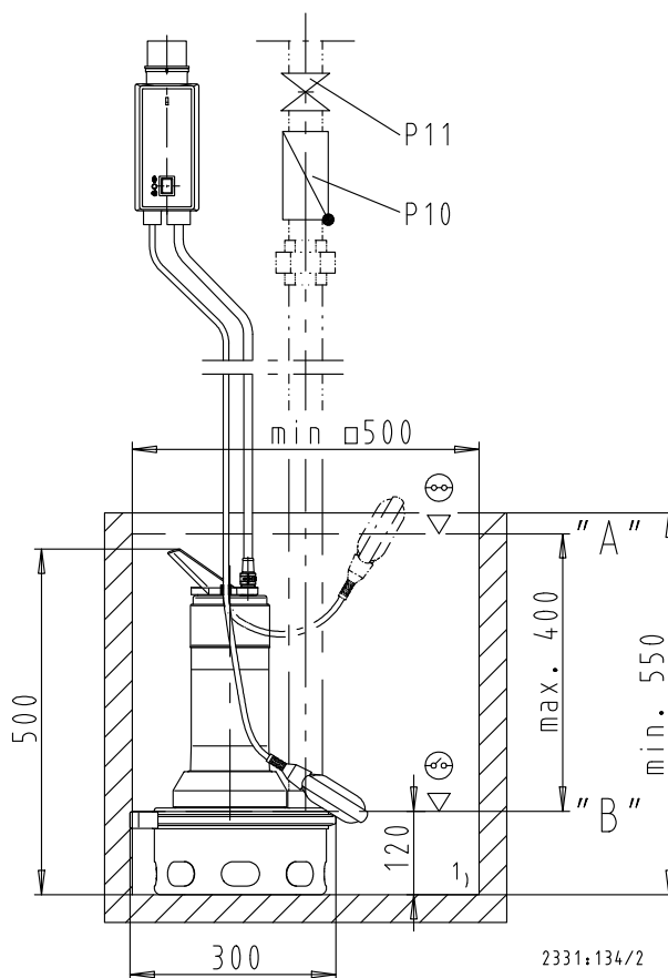
III. 6: AmaDrainer 4, pompe simple, passage libre 35 mm, avec interrupteur à flotteur, moteur triphasé, sans enveloppe de refroidissement
